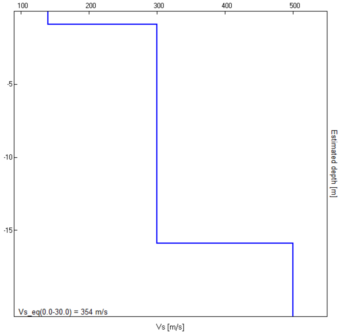
FIG. 5 - MODELLO STRATIGRAFICO-SISMICO
