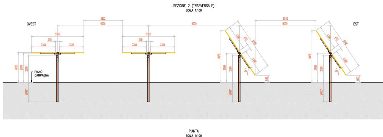
Particolare strutture sostegno moduli pannelli e distanze di campo (interfila m 9,0)
