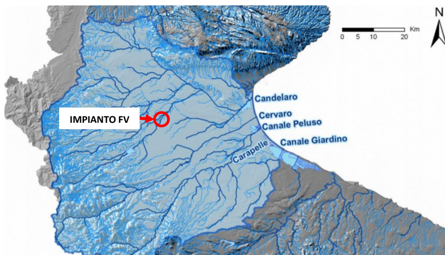
Figura 3.5: Corpi idrici superficiali (Relazione PGRA - AdB Puglia) ed ubicazione area di progetto.
