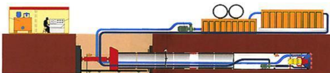
Schematico di Perforazione con Microtunneling
