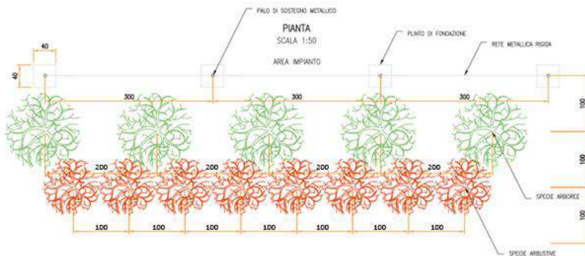
Figura 2.75: Tipologico filare di mitigazione
