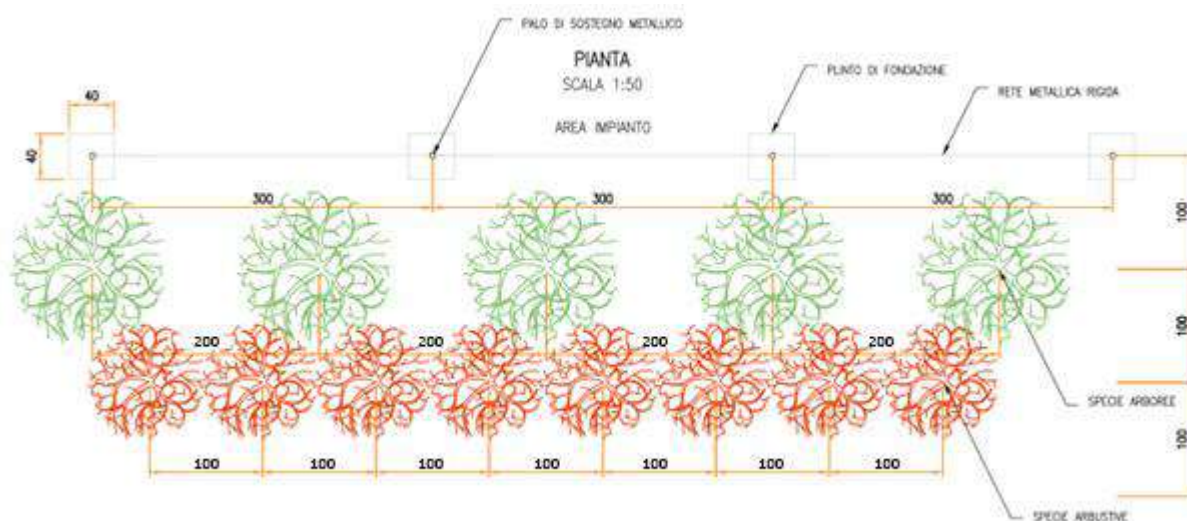
Figura 4.121: Tipologico del filare di mitigazione
