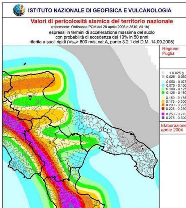
Figura 4.63: Carta della pericolosità sismica della Puglia.
