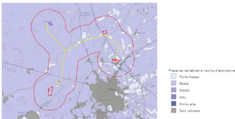
Figura 4.41: Carta della Natura della Regione Puglia (fonte: ISPRA Dati del Sistema Informativo di Carta della Natura – Lavarra, 2014): Presenza vertebrati a rischio d'estinzione
