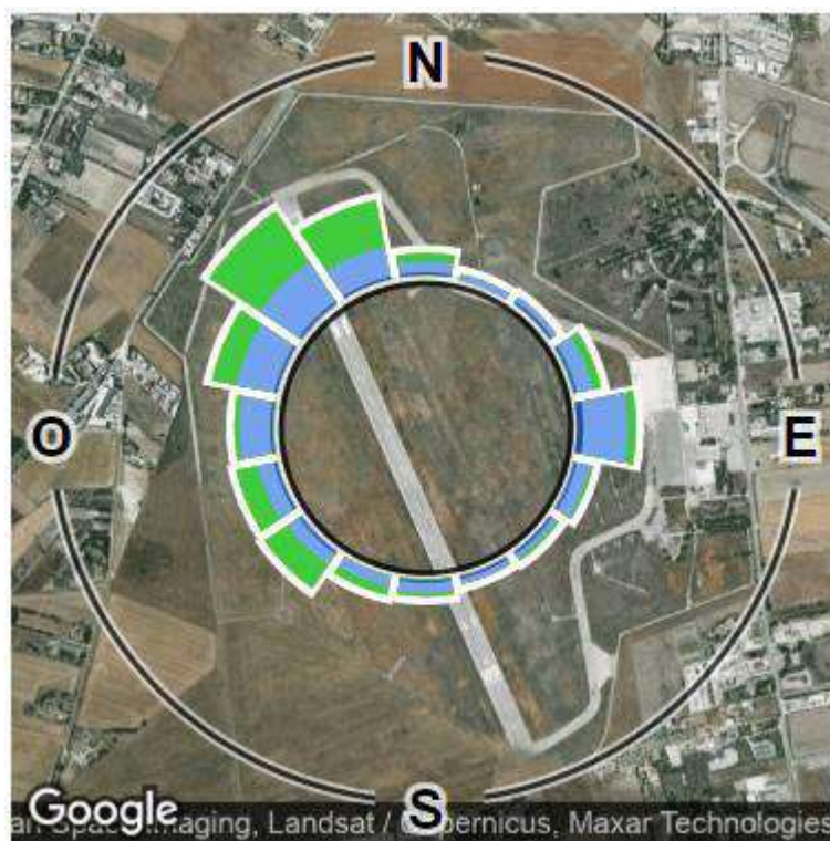
Figura 4.83: Rosa dei venti nell'area di Foggia nel periodo 2002 – 2019
