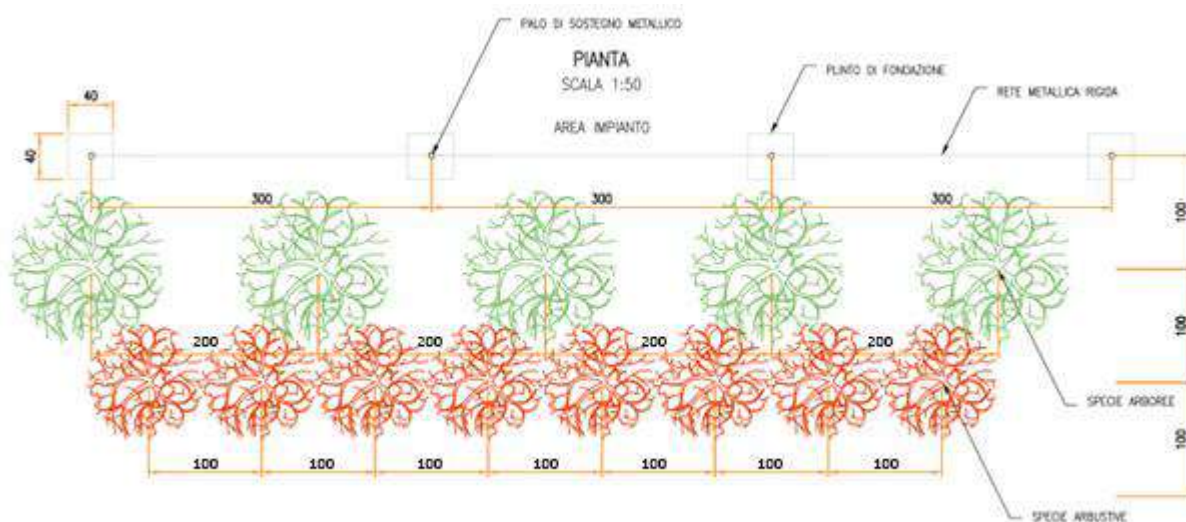
Figura 2.68: Tipologico filare di mitigazione
