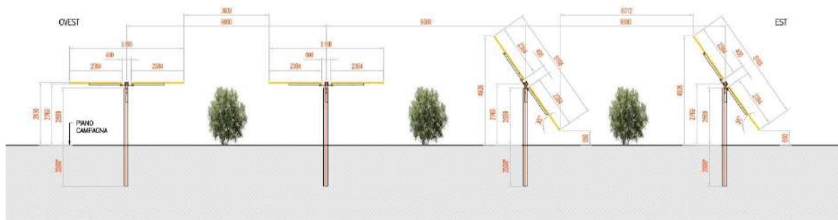
Figura 2.70: Tipologico – Sezione dell'impianto Olivicolo.
