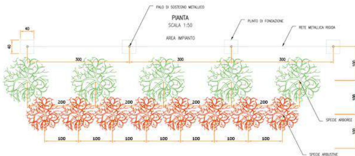
Figura 2.56: Tipologico del filare di mitigazione
