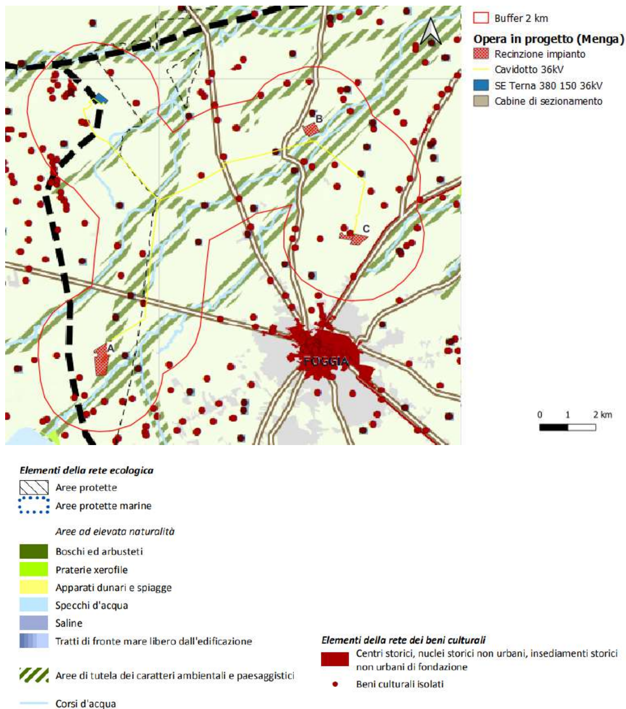
Figura 4.26: Schema della Rete Ecologica Provinciale della Provincia di Foggia con dettaglio all'interno del buffer di 2 km – fonte: PTCP Foggia (Tavola S1 - Il sistema delle qualità)
