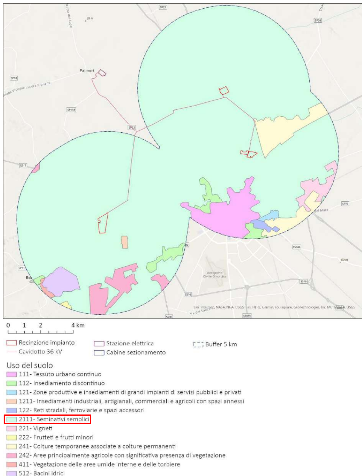
Figura 4.21: Uso del suolo nel buffer di 5 Km intorno all'area di previsto intervento. Fonte: Corine Land Cover (ISPRA).
