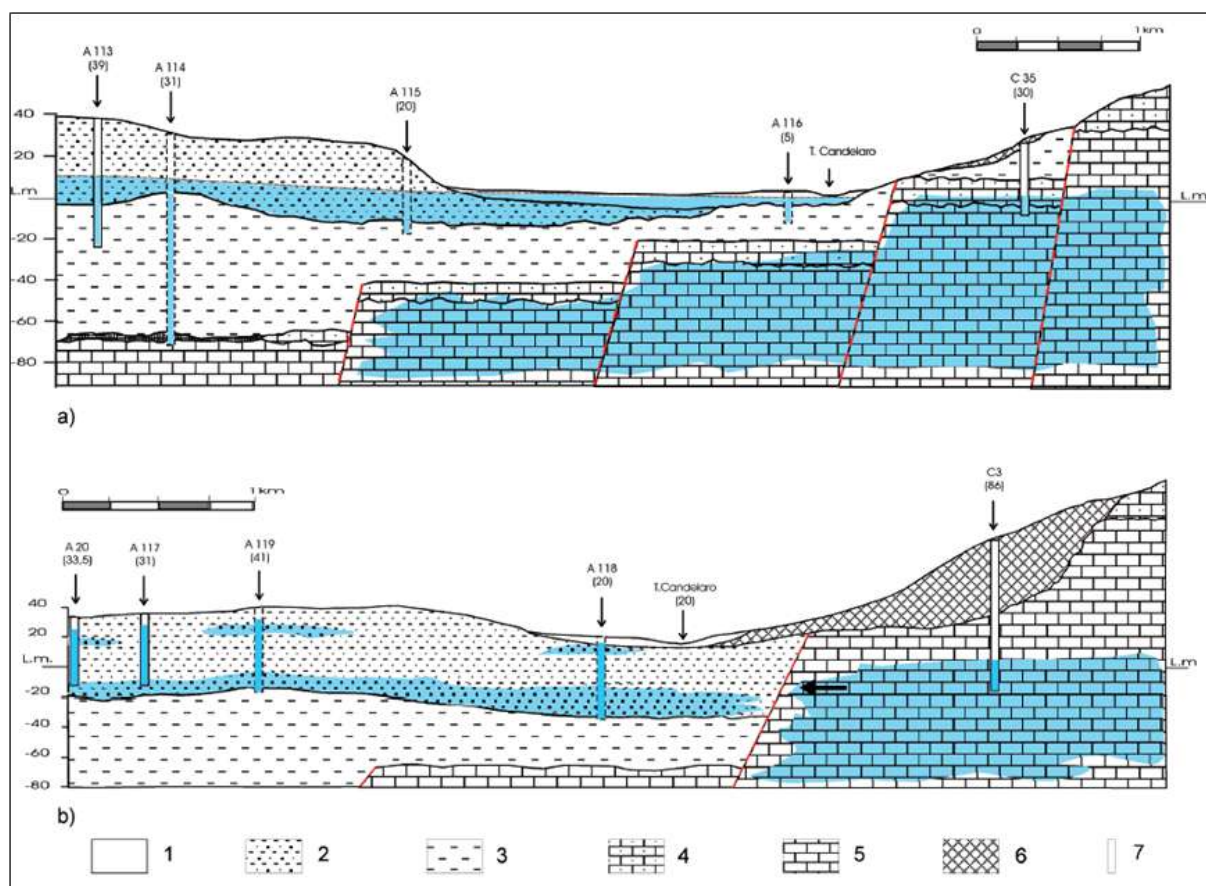
Figura 4.61: Sezioni idrogeologiche. Legenda 1) Depositi d'alveo (Olocene); 2) depositi della pianura alluvionale (Olocene – Pleistocene sup.); 3) argille grigio- azzurrognole con intercalazioni sabbiose (Pleistocene inf. – Pliocene sup.)
