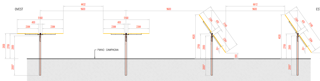
• Figura 4.6: Particolare strutture di sostegno moduli
