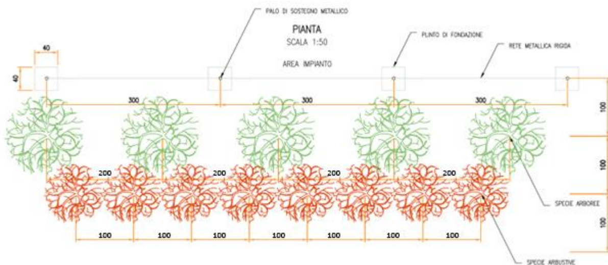
• Figura 5.4: Tipologico del filare di mitigazione
