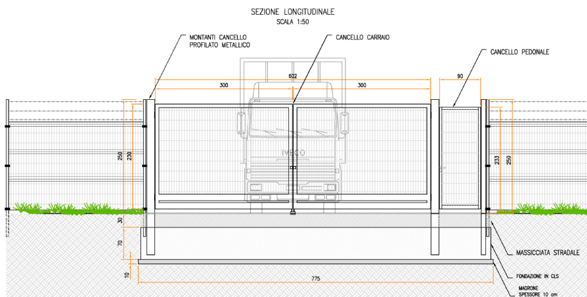
• Figura 4.9: Particolare accesso
