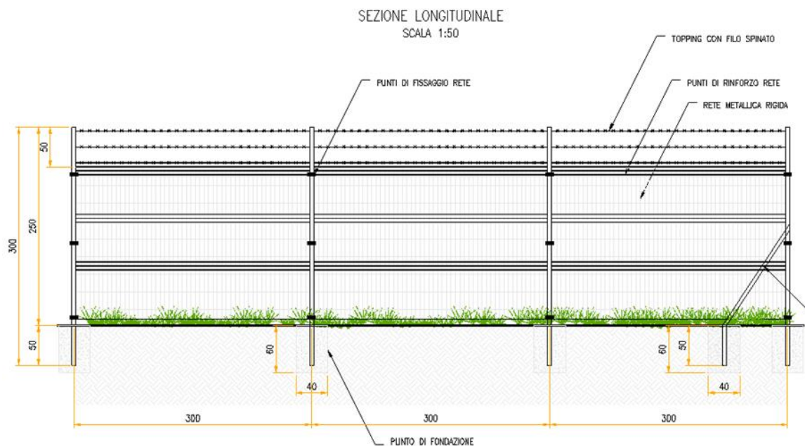
• Figura 4.7: Particolare recinzione
