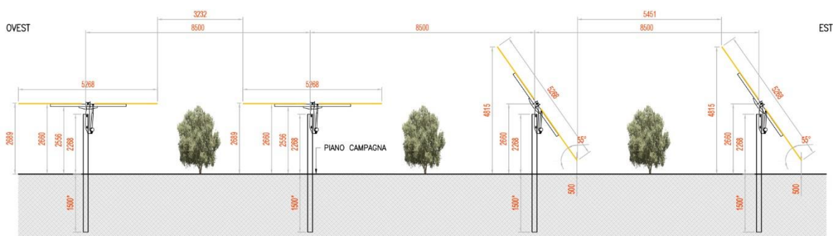
Figura 6.4: Tipologico – Vista Planimetrica dell'impianto Olivicolo
