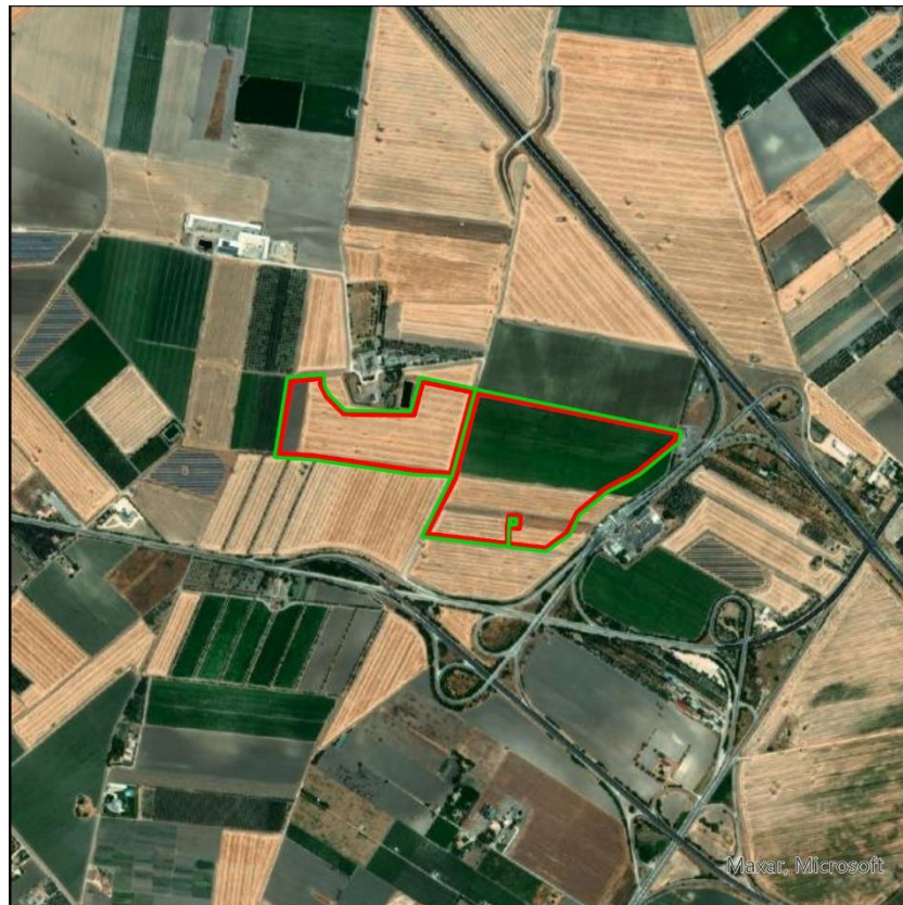
• Figura 5.2: Localizzazione delle Opere a Verde di mitigazione – Area Centro
