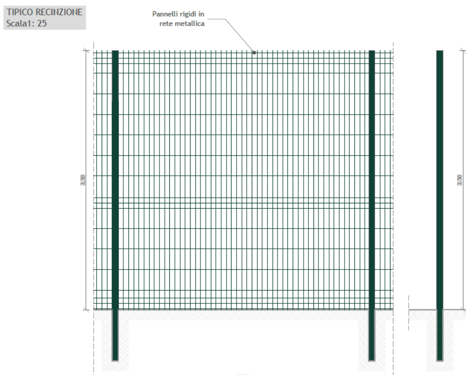
Figura 10. Dettaglio costruttivo della recinzione
