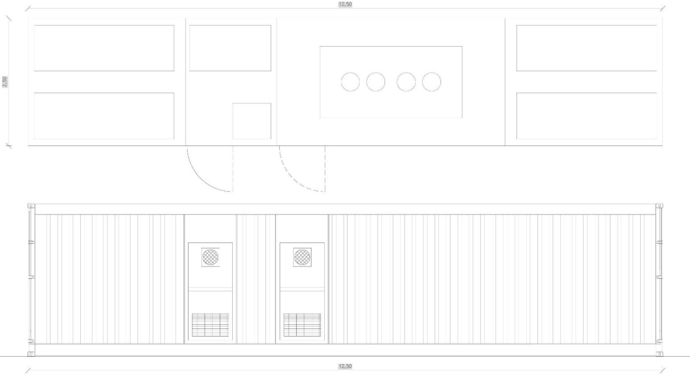
Figura 8. Pianta e prospetto della cabina PCS
