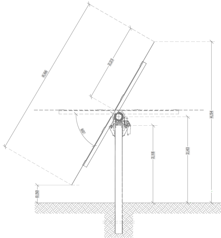
Figura 4. Particolare costruttivo
