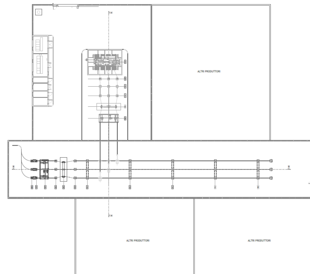
Planimetria Elettromeccanica
