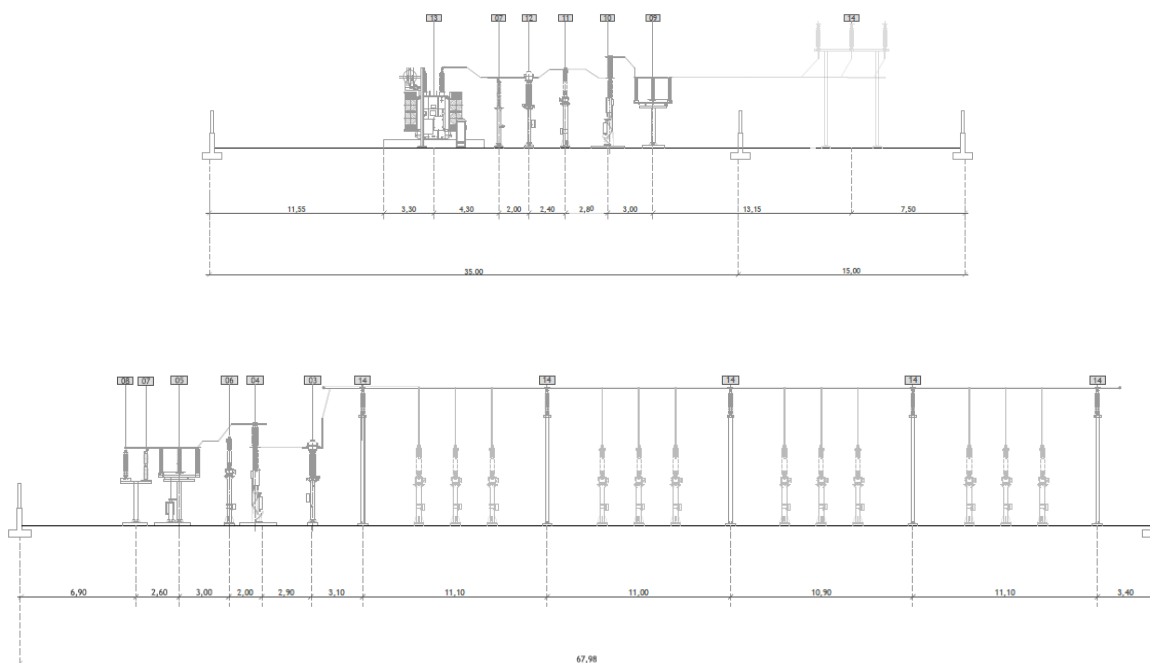
Sezioni Elettromeccaniche
