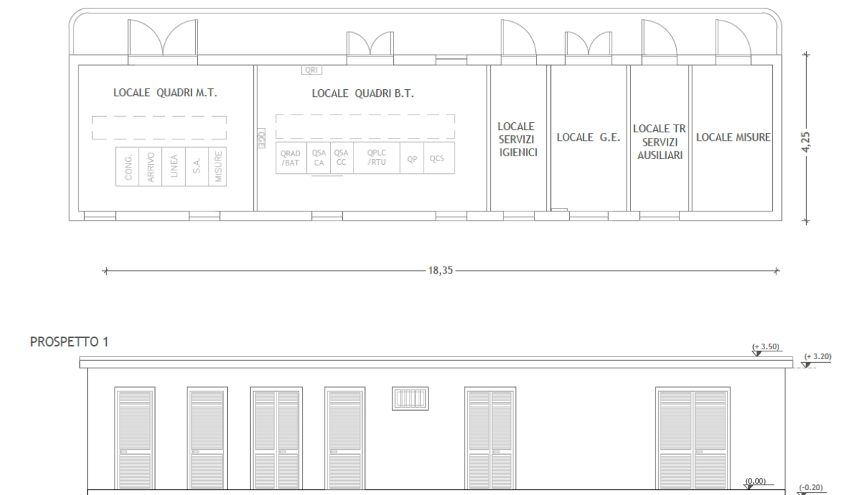
Fig. Pianta e prospetto edificio
