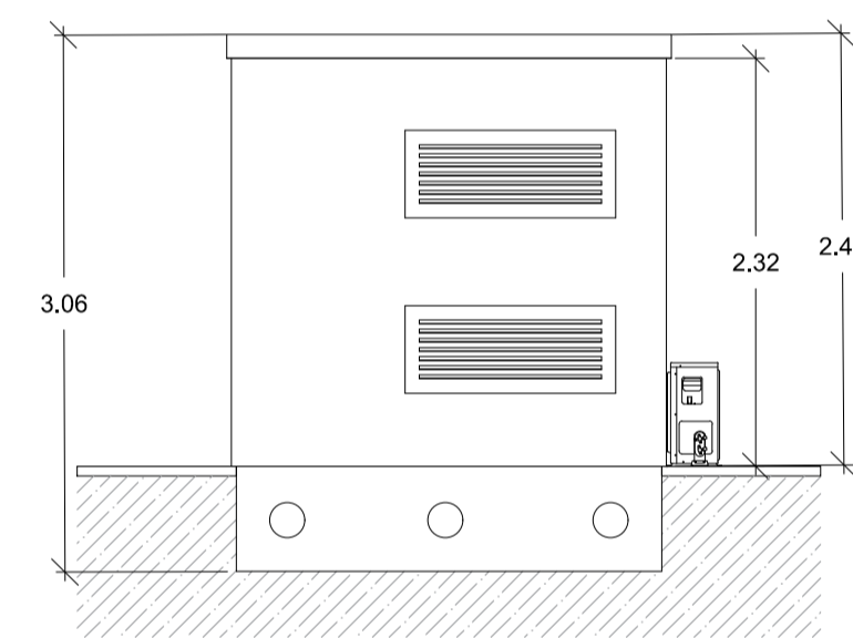
VISTA LAT. DX
