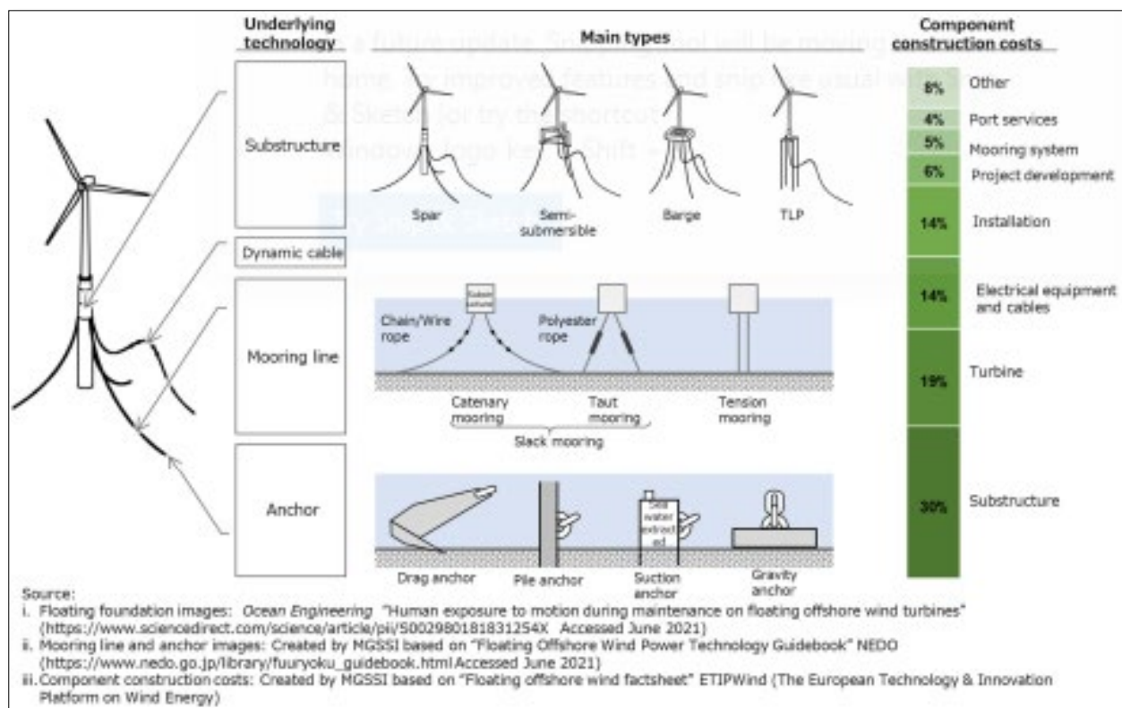
Figura 2.2: Tecnologie per l'energia eolica offshore galleggiante
