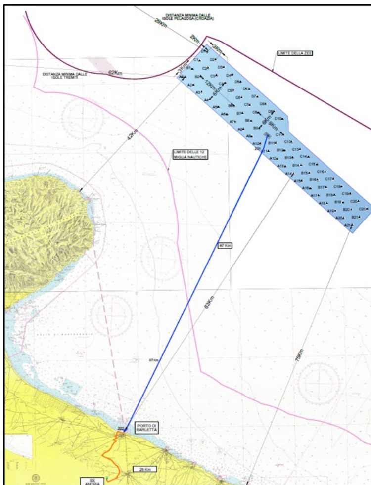
Figura 2: Layout impianto su carta nautica di dettaglio.
