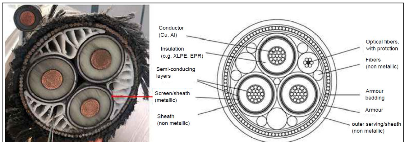
Figura 6: Struttura cavo 66 kV.
