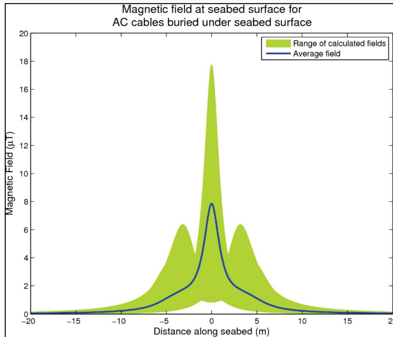
Figura 13: Diagramma dell'intensità del campo magnetico generato sulla superficie del fondo marino da cavo AC sepolto
