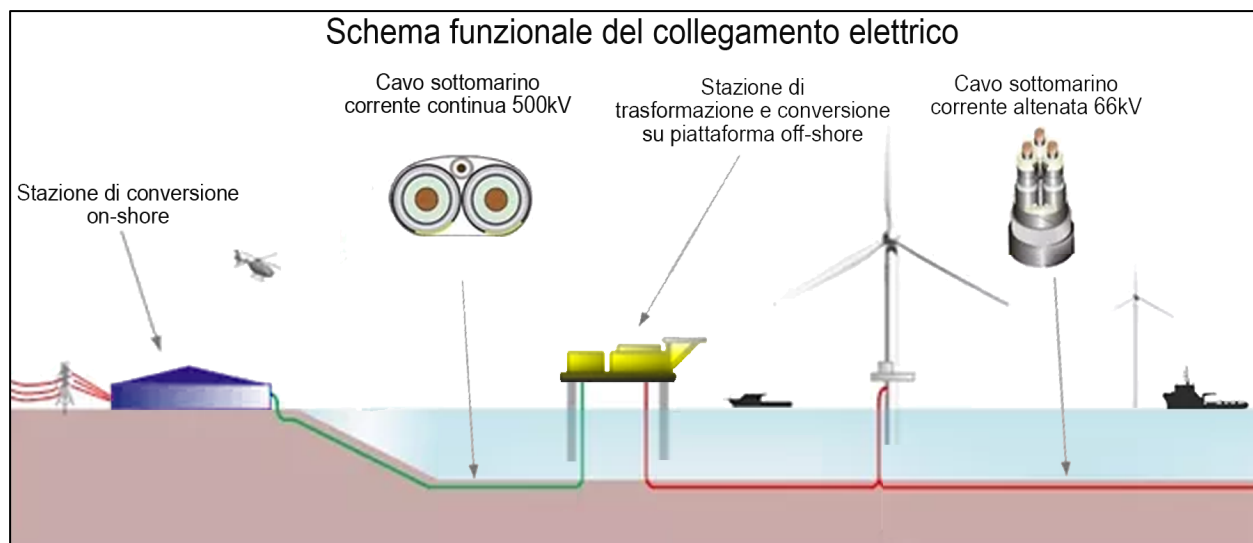
Figura 7: Schema funzionale di collegamento elettrico.
