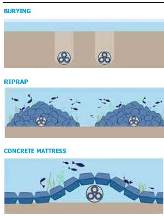
Figura 10: Tecniche principali di posa dei cavi sottomarini (da Normandeau et al., 2011)
