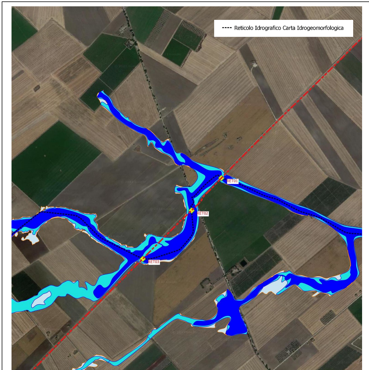
Figura 6 – Cavidotto di vettoriamento e interferenze con reticolo idrografico (da RET01 a RET03) e fasce a pericolosità idraulica del PAI Puglia (aggiornamento 2019)
