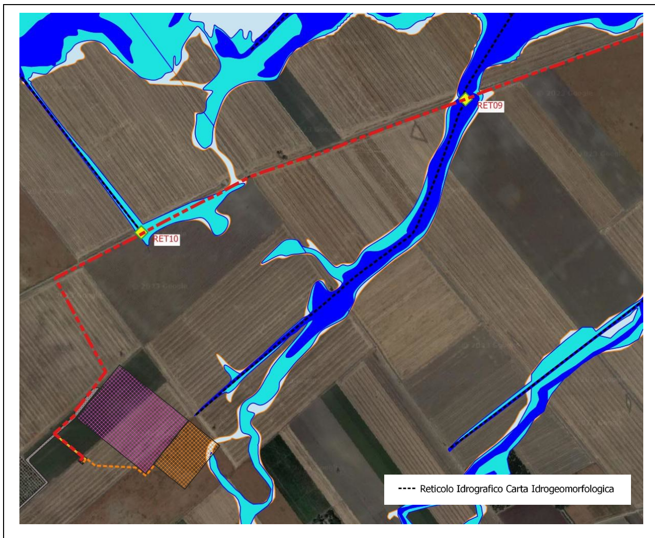
Figura 8 – Cavidotto di vettoriamento e interferenze con reticolo idrografico (da RET09 a RET10) e fasce a pericolosità idraulica del PAI Puglia (aggiornamento 2019)
