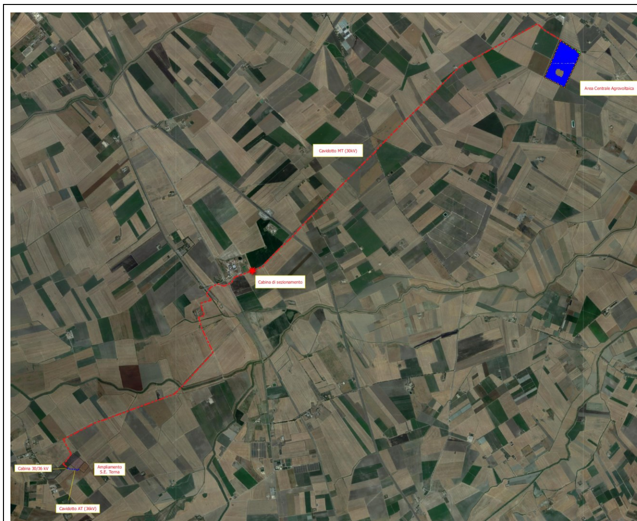
Figura 1 – Centrale agrovoltaica e infrastrutture connesse
