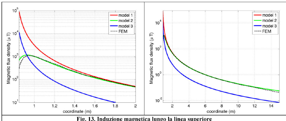
Fig. 13. Induzione magnetica lungo la linea superiore
