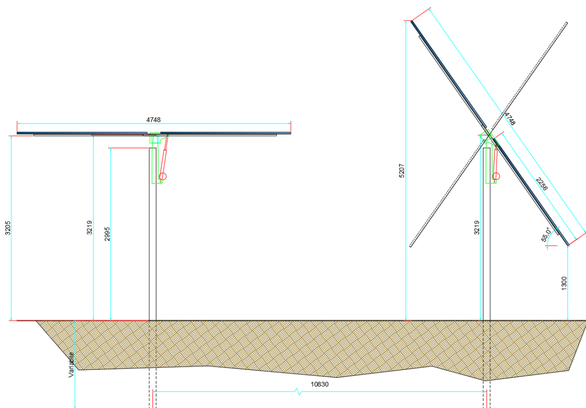
Fig. 2- Tracker - Inseguitore mono-assiale - intervalli di rotazione
