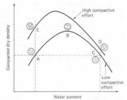
Figura 49 Curva di compattazione in terreni coerenti
