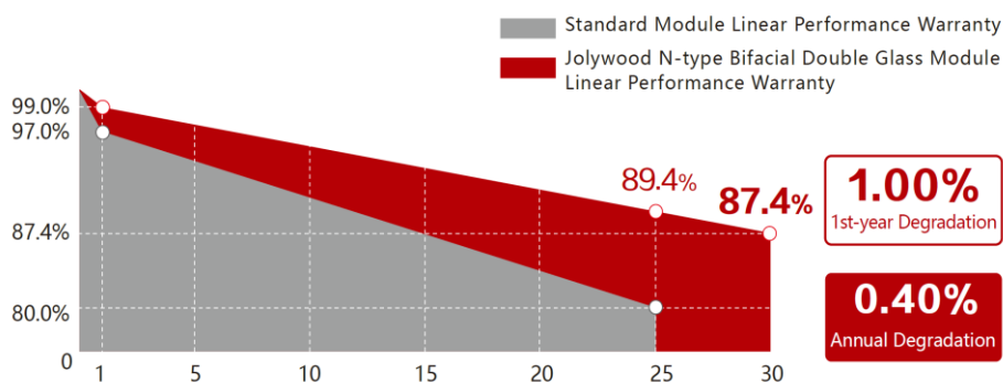
Figura 7 - variazione rendimento dei pannelli col tempo
