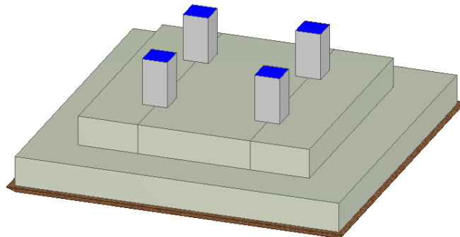
Fig. Vista assonometrica fondazione per palo gatto
