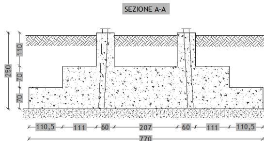
Fig. Pianta e sezione fondazione per palo gatto
