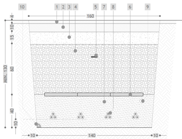
Figura 2: Sezione tipo cavidotto MT composta da quattro terne una da 400 e tre da 630 mm 2
