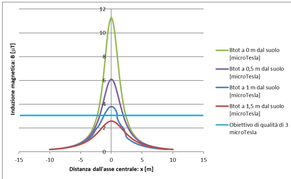
Figura 3: Andamento del campo magnetico generato dal cavidotto MT, composta da quattro terne una da 400 e tre da 630 mm 2
