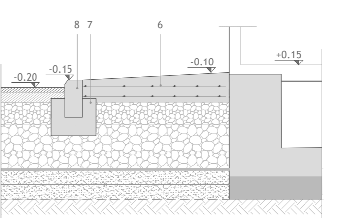
Dettaglio marciapiede Scala 1: 25
