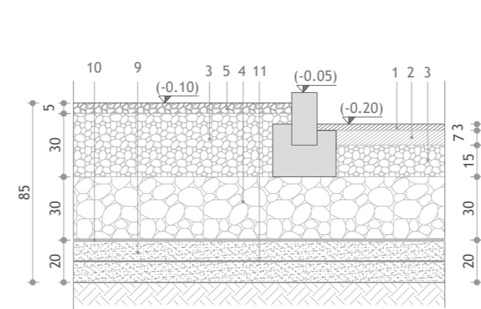
Dettaglio Viabilità / Piazzali Scala 1: 25
