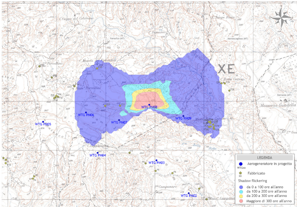
Figura 9 - Mappa di impatto potenziale per l'aerogeneratore WTG PM08
