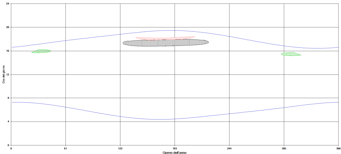
Figura 13 – Calendario dell'ombra nelle condizioni caso peggiore per il fabbricato 24
