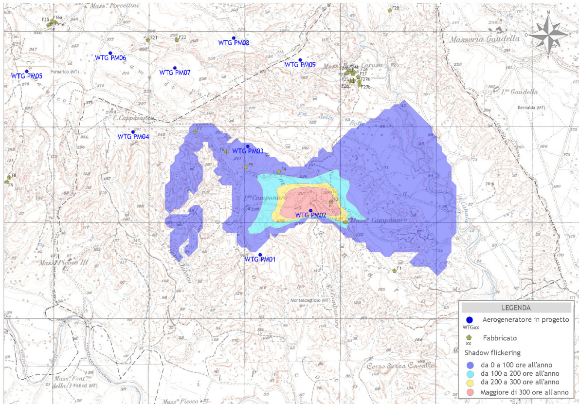
Figura 3 - Mappa di impatto potenziale per l'aerogeneratore WTG PM02
