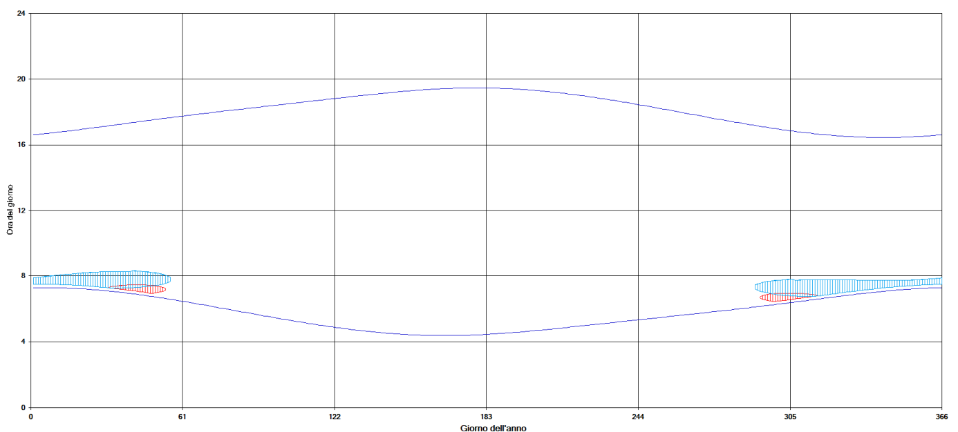
Figura 12 – Calendario dell'ombra nelle condizioni caso peggiore per il fabbricato 16
