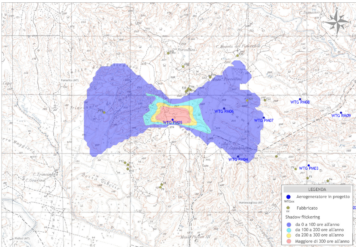
Figura 6 - Mappa di impatto potenziale per l'aerogeneratore WTG PM05
