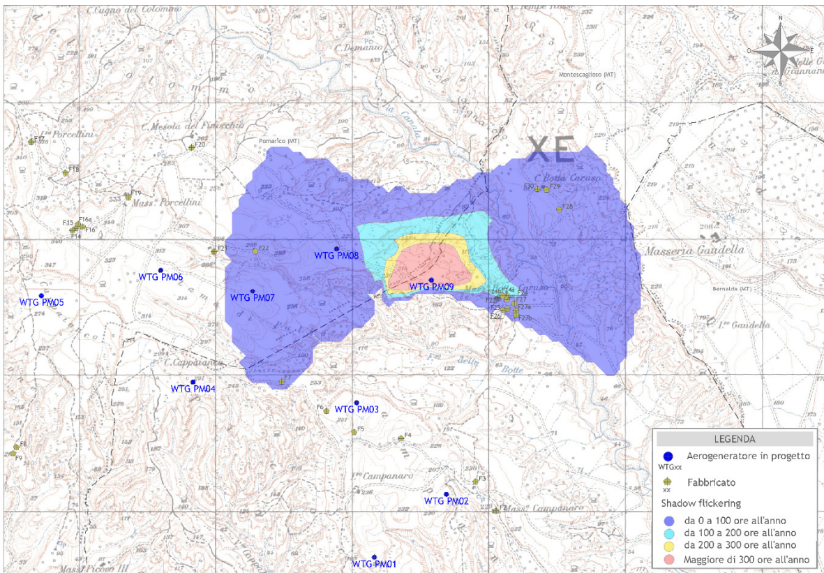
Figura 10 - Mappa di impatto potenziale per l'aerogeneratore WTG PM09
