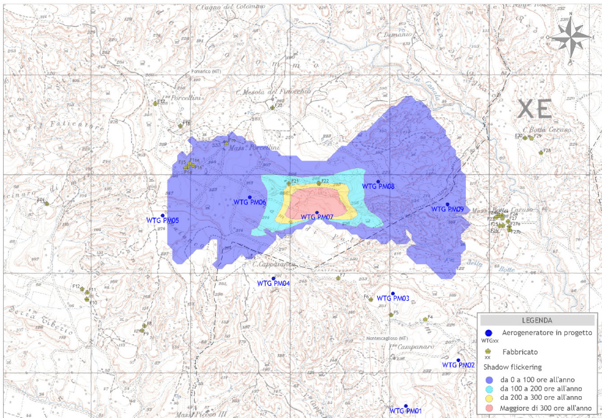
Figura 8 - Mappa di impatto potenziale per l'aerogeneratore WTG PM07
