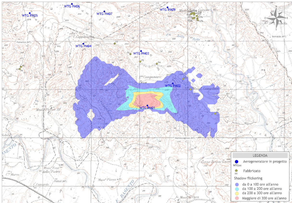
Figura 2 - Mappa di impatto potenziale per l'aerogeneratore WTG PM02
