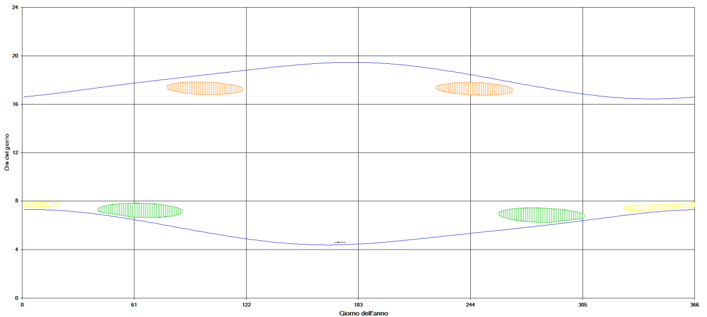
Figura 11 – Calendario dell'ombra nelle condizioni caso peggiore per il fabbricato 7
