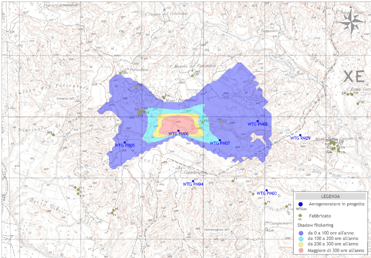
Figura 7 - Mappa di impatto potenziale per l'aerogeneratore WTG PM06
