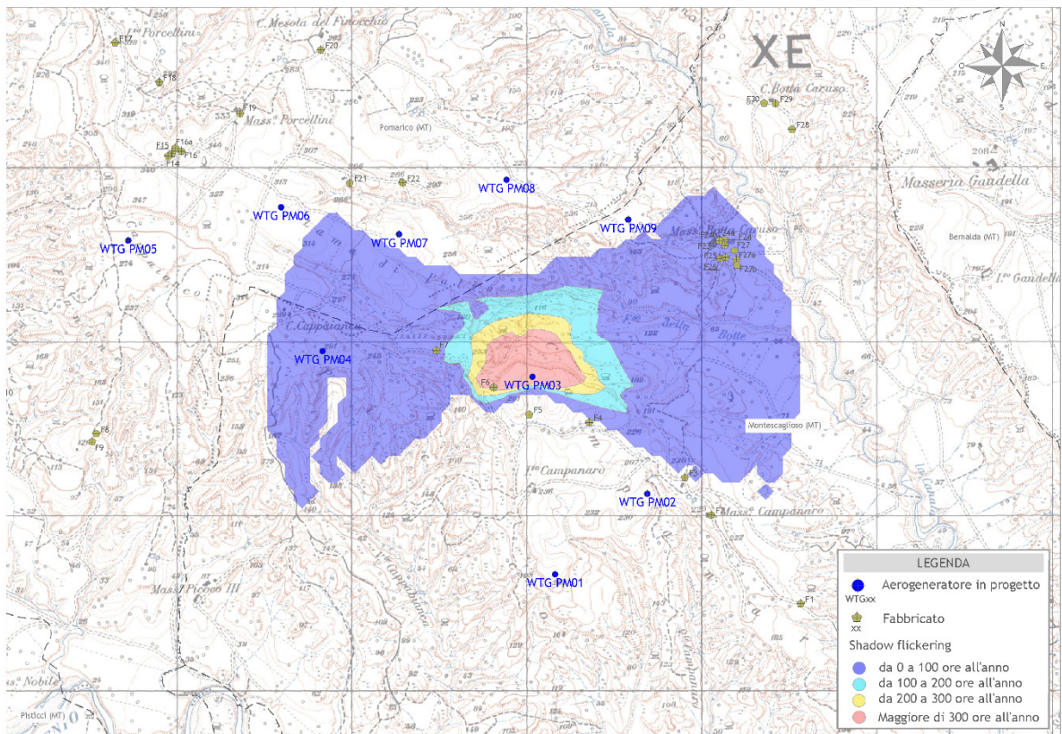
Figura 4 - Mappa di impatto potenziale per l'aerogeneratore WTG PM03
