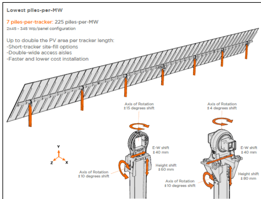
Figura 9 – schema tipo funzionamento inseguitore monoassiale
