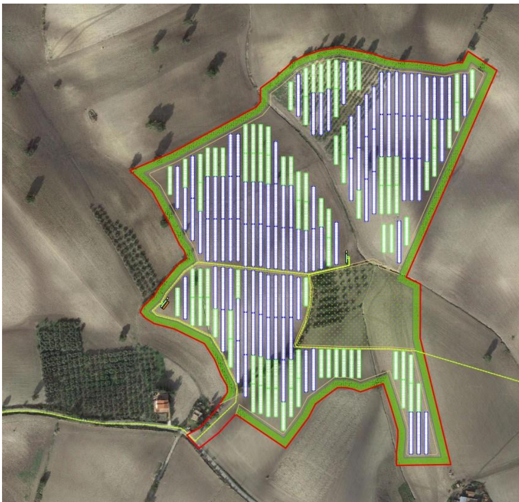
Figura 7 - Layout impianto Plot 2
