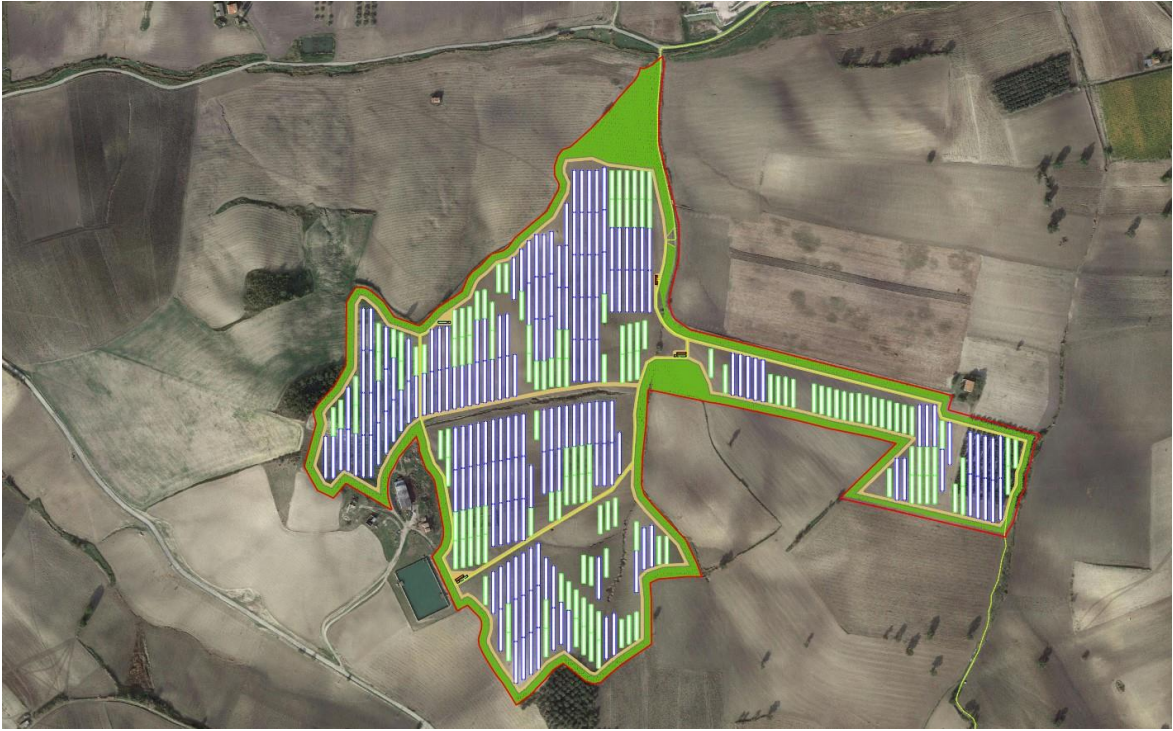
Figura 6 - Layout impianto Plot 1
