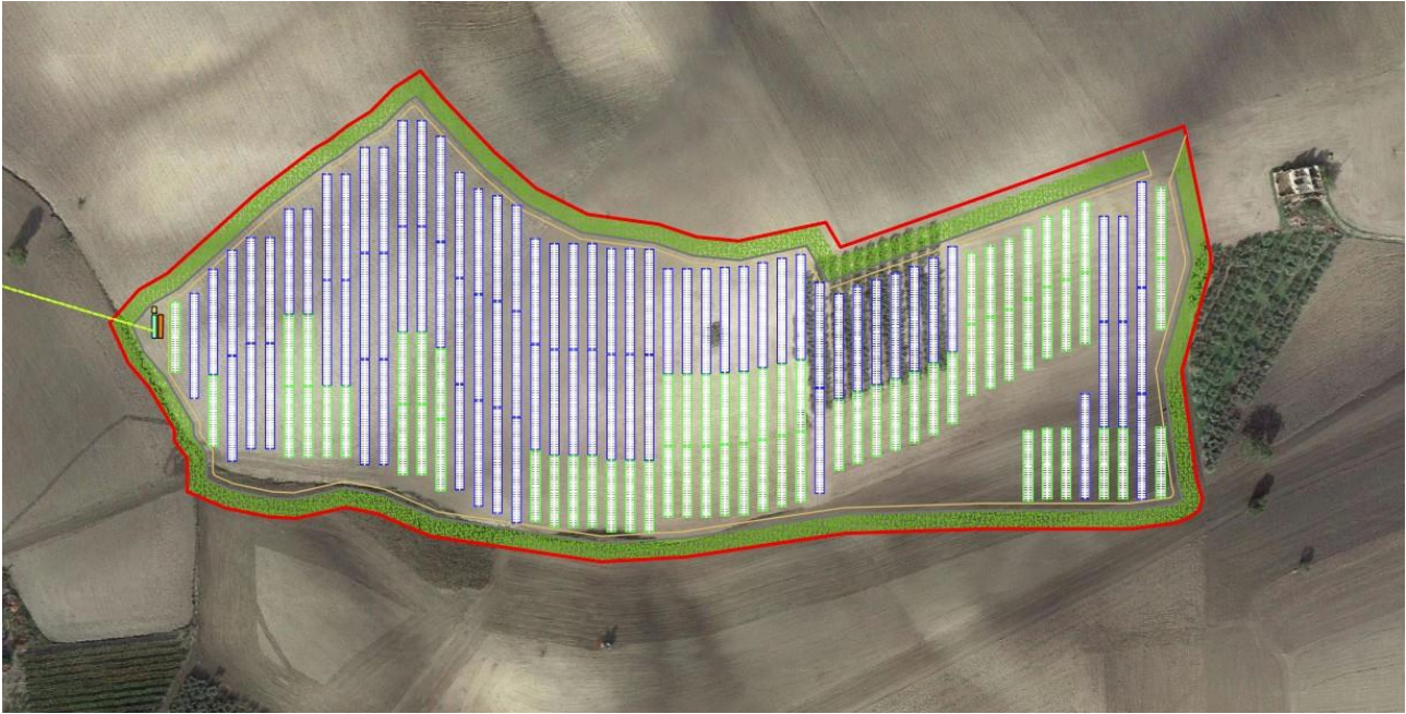
Figura 8 - Layout impianto Plot 3
