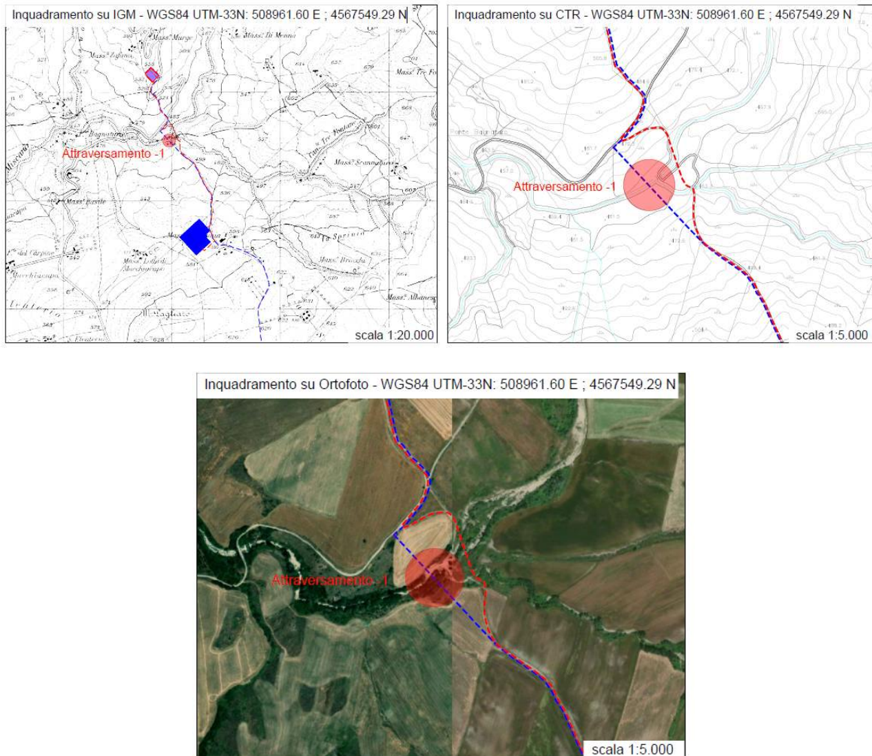
Figura 11 Inquadramento su IGM, Ortofoto, CTR e Catastale dell' interferenza con il Fiume vincolato "Miscano" e Attraversamento n.1 tramite TOC (cfr. Tavola degli attraversamenti)
