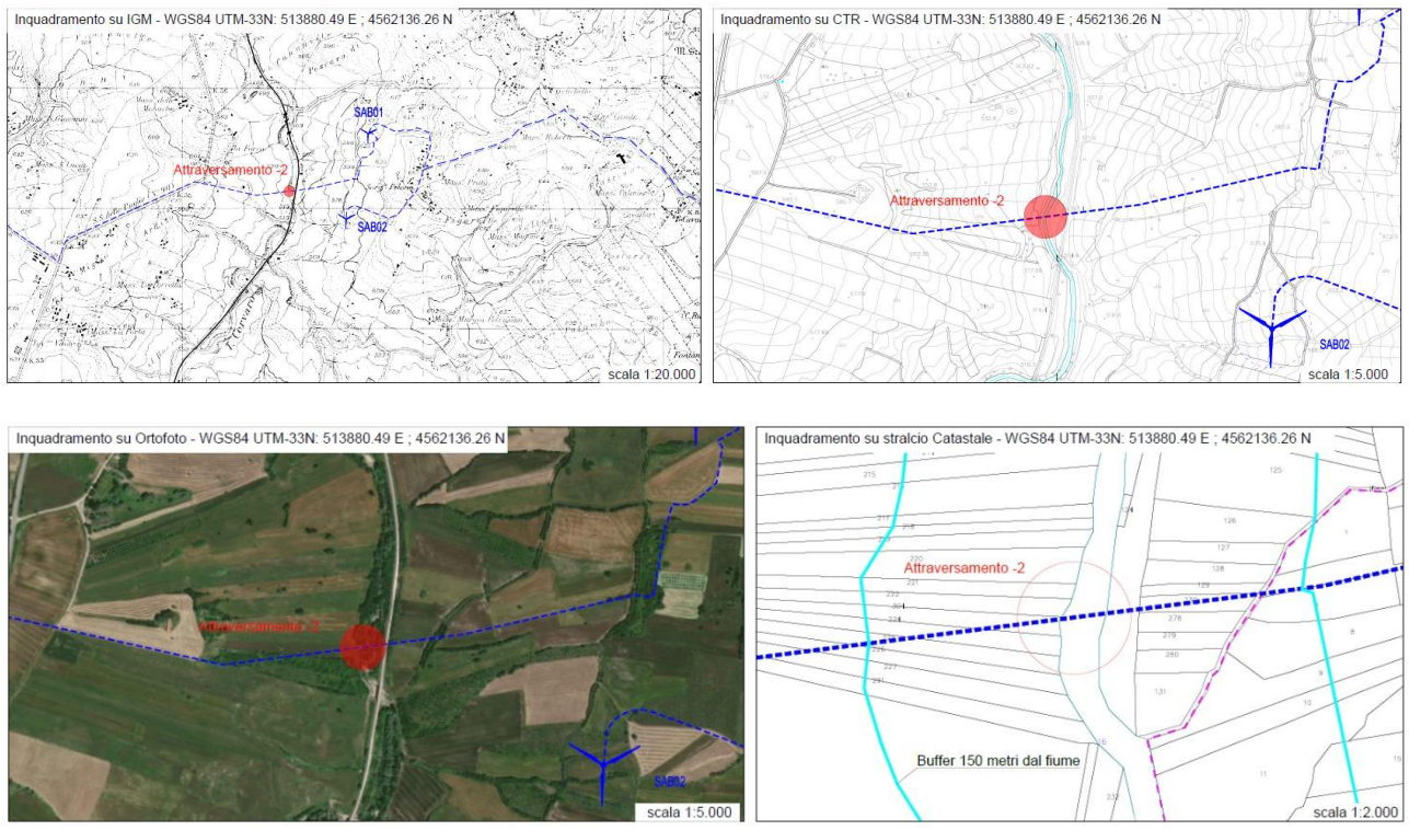
Figura 9 Inquadramento su IGM, Ortofoto, CTR e Catastale dell' interferenza con il Fiume vincolato "Cervaro" e Attraversamento n.2 tramite TOC (cfr. Tavola degli attraversamenti)
