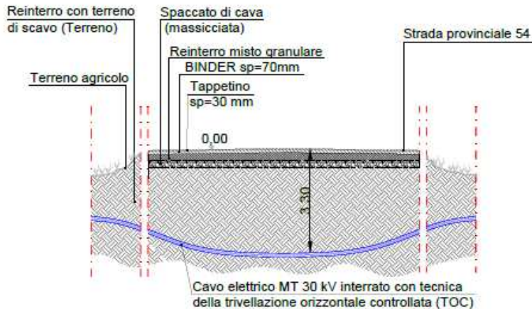
Figura 15 Tipico attraversamento TOC su strada
