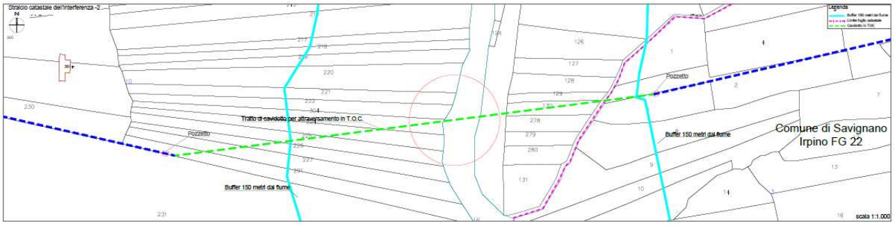
Figura 10 Attraversamento N.2 in TOC (cfr. Tavola degli attraversamenti)
