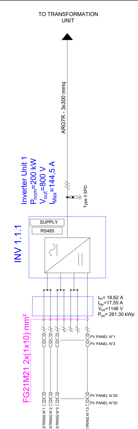
Tipologico collegamento Stringhe e String Box
