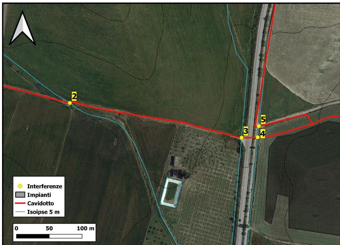
Figura 3: Dettaglio delle interferenze 2, 3, 4 e 5 su CTR. Base cartografica: Google Satellite.
