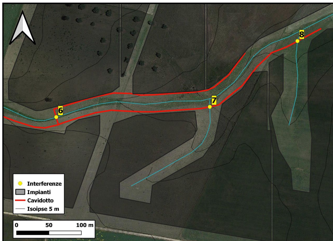
Figura 4: Dettaglio delle interferenze 6, 7, e 8 su CTR. Base cartografica: Google Satellite
