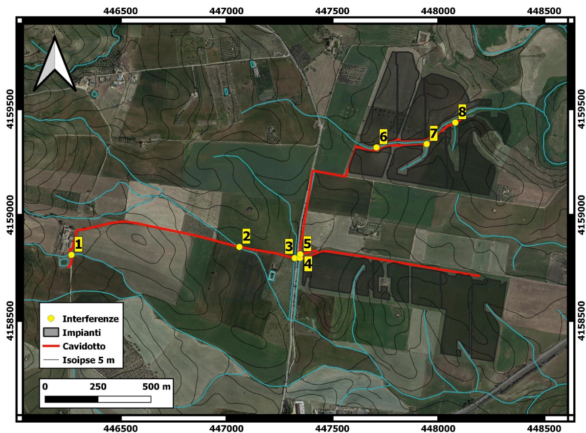
Figura 1: Localizzazione opere di progetto su cartografia CTR 1:10000 e relative interferenze con il reticolo idrografico su mappa base Google Satellite. Coordinate in WGS84 – UTM 33N.
