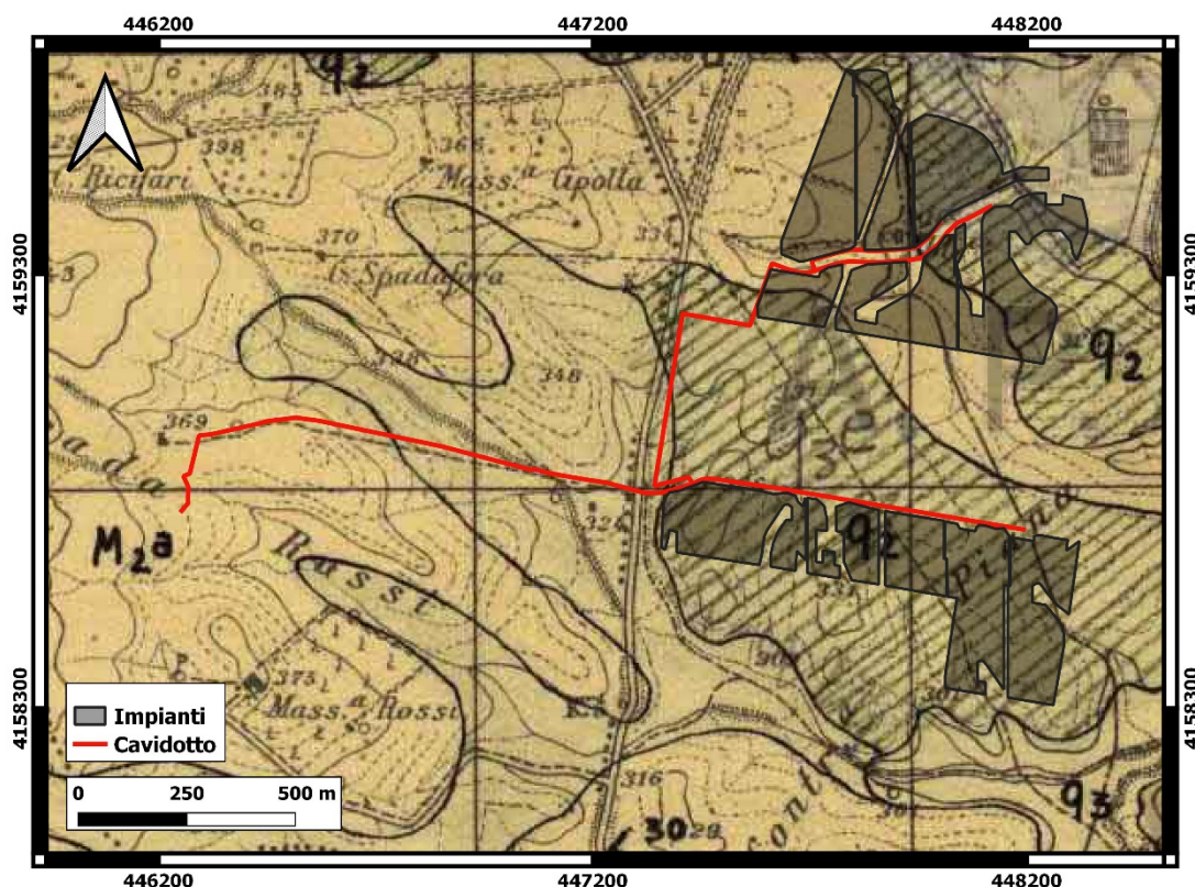
Figura 2: Carta geologica redatta dall’Agenzia per la protezione dell’ambiente e per i servizi tecnici (APAT). La sigla M2a identifica la Formazione di Terravecchia, la q2 i depositi fluviali antichi collegabili con l’idrografia attuale e la q3 i depositi fluviali antichi indipendenti dall’idrografia attuale. Coordinate in WGS84 – UTM 33N.
