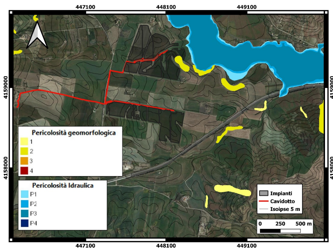
Figura 4: Carta della pericolosità geomorfologia ed idraulica secondo il P.A.I. Coordinate in WGS84 – UTM 33N.
