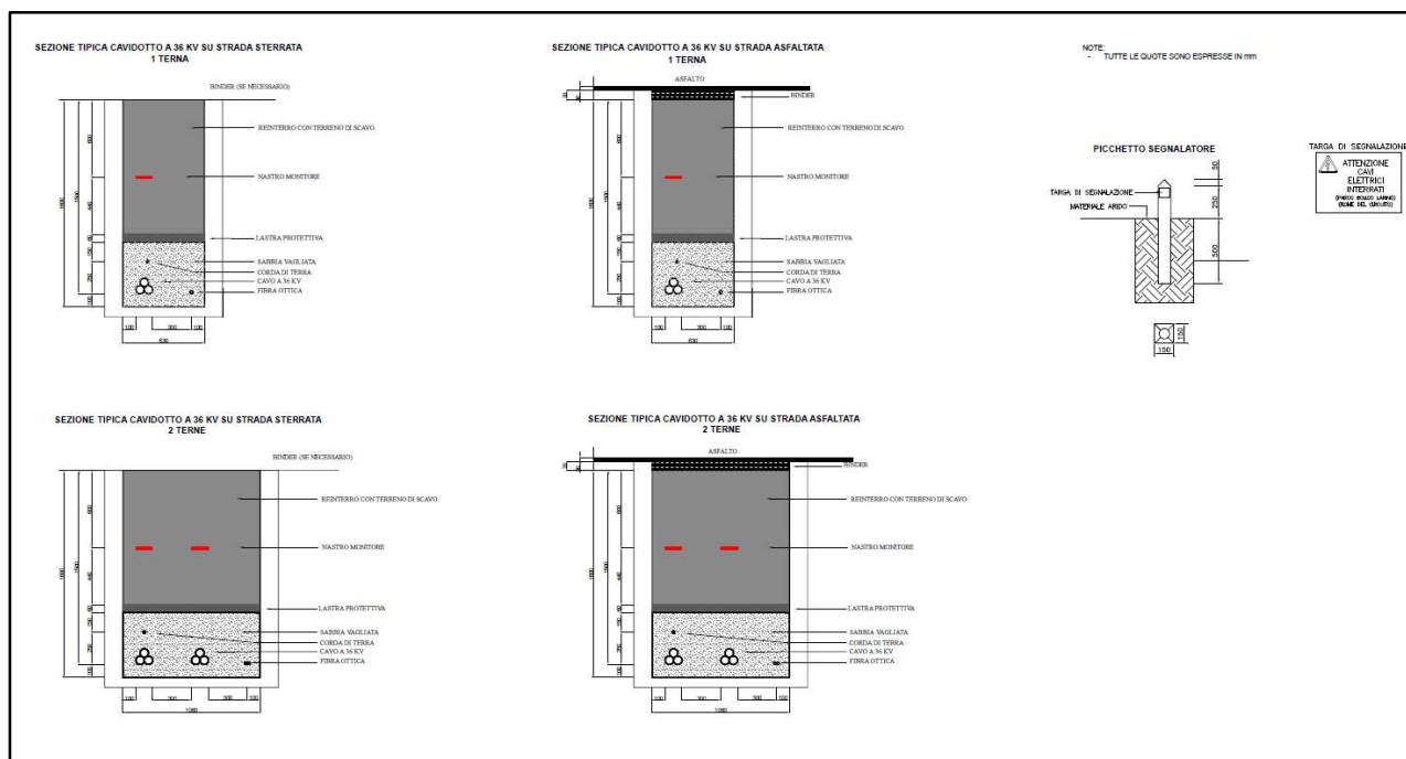
Figura 2.3.1.1: Sezioni tipiche delle trincee caavidotto per una o due terne di cavi in parallelo
