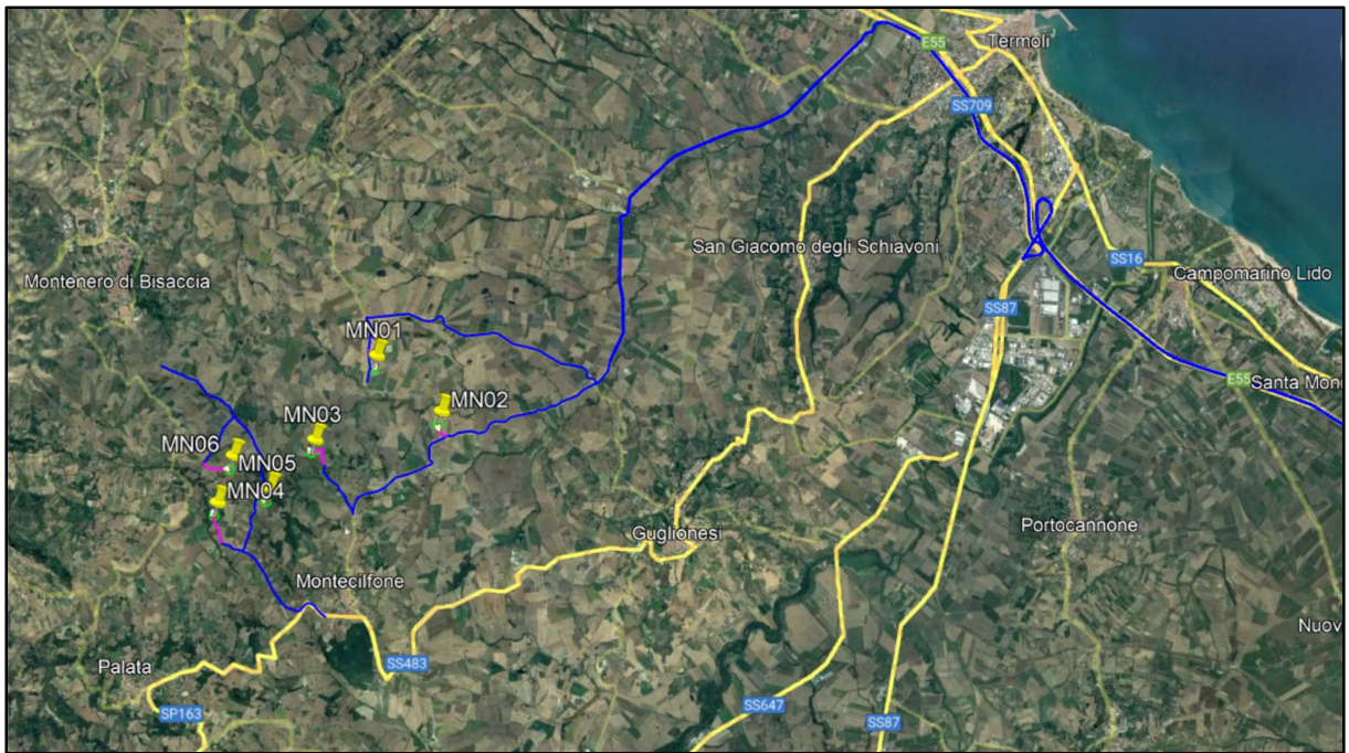
Figura 6.3: Layout d’impianto con sistema di viabilità esistente (linee blu) e di progetto (linee magenta) su immagine satellitare
