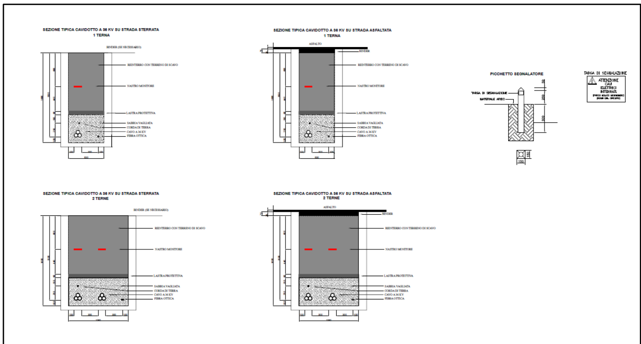
Figura 3.3.2.1: Sezioni tipiche delle trincee caavidotto per una o due terne di cavi in parallelo
