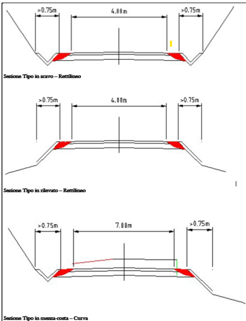
Figura 3.2.1: Sezioni tipo viabilità parco eolico
