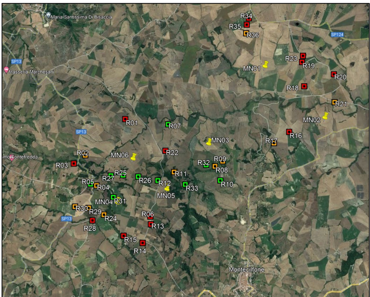
Figura 7.2.1: Localizzazione dei fabbricati nell'area d'impianto e degli aerogeneratori di progetto
