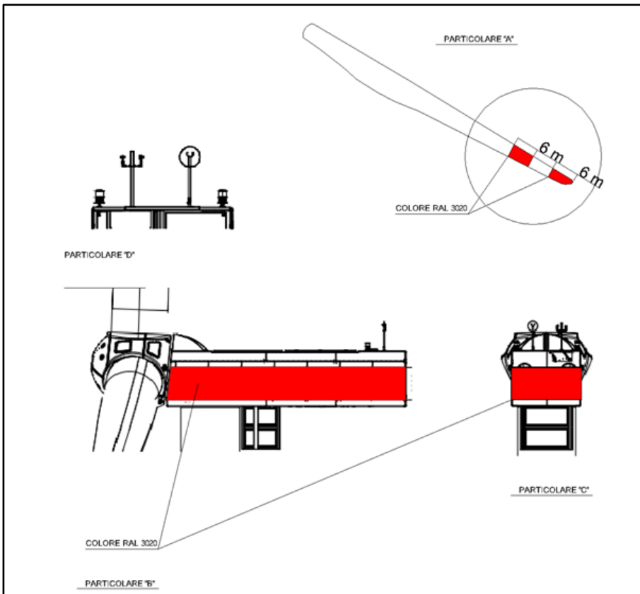
Figura 3.1.2: Particolari aerogeneratore SG170 – 6.0 MW
