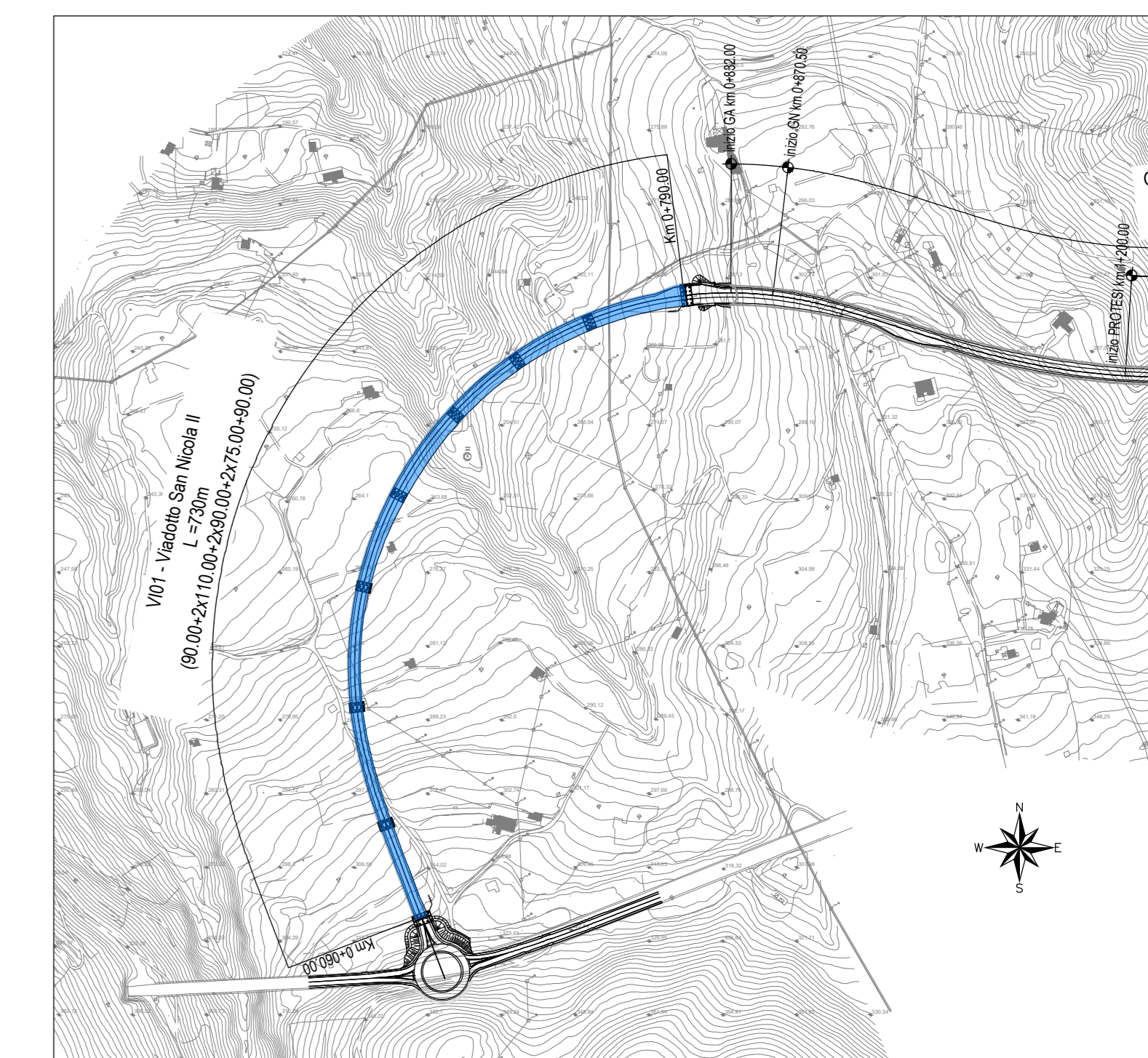
STRALCIO PLANIMETRICO scala 1:5000
