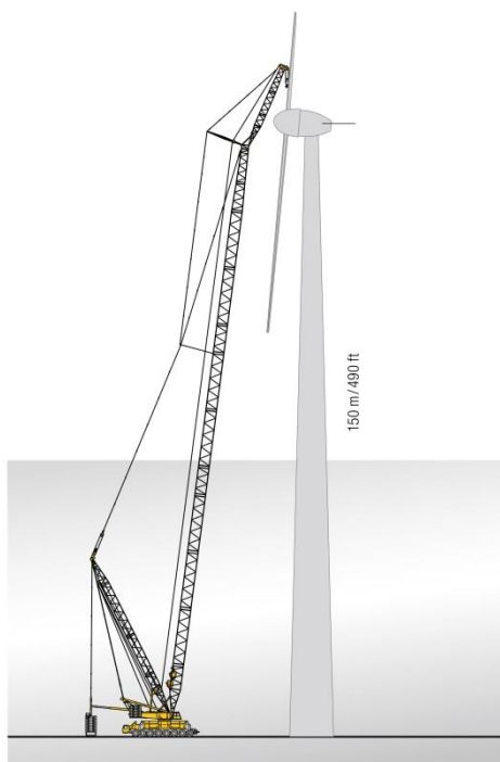
Figura 5-28 – Schema di una gru cingolata a traliccio con sistema derrick impiegata per l'innalzamento delle turbine eoliche dell'ultima generazione
