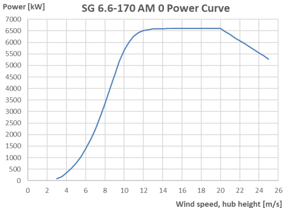
Figura 4-1 - Curva di potenza generatore tipo SG 6.6-170
