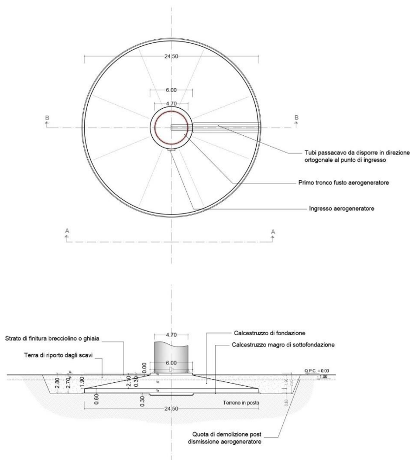
Figura 5-29 – Pianta e vista della fondazione tipo dell'aerogeneratore
