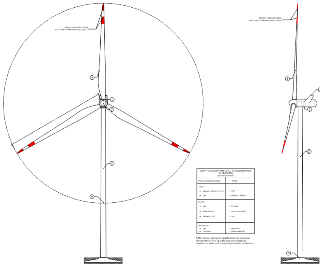
Figura 4-3 – Aerogeneratore tipo SG 6.6-170 altezza al mozzo (1) 125m, e diametro rotore (2) di 170m
