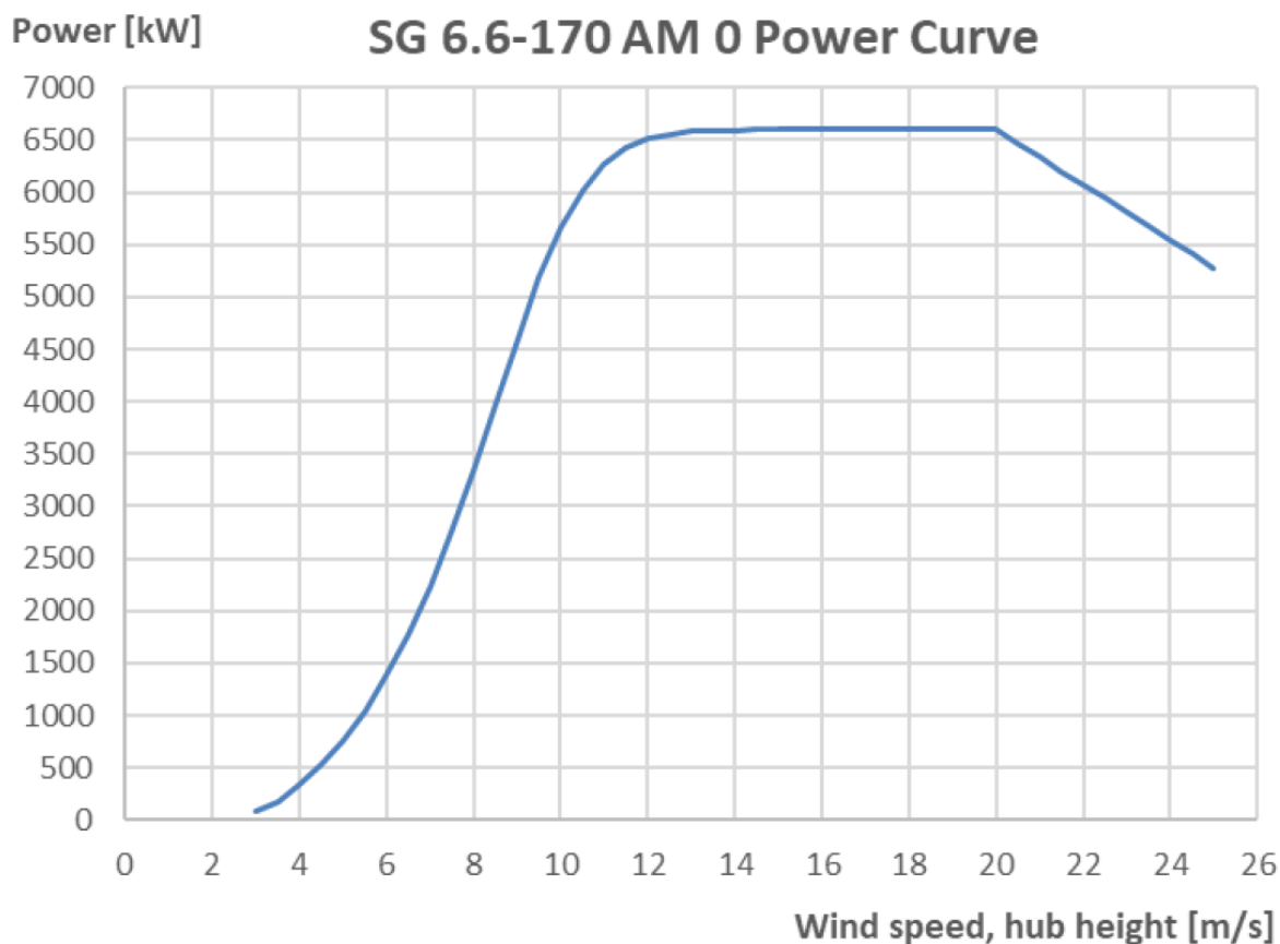
Figura 3-3 - Curva di potenza generatore tipo SG 6.6-170
