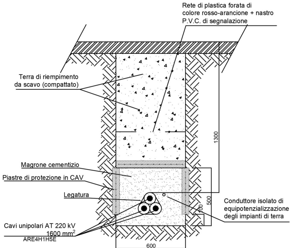
Figura 3-6 - Modalità di posa Cavo AT 200/345 kV
