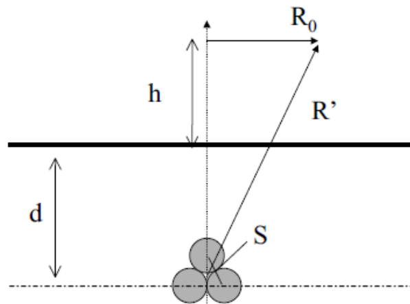
Figura 8-1 - Schema di principio per il calcolo delle distanze da terne di cavi interrati con posa a trifoglio oltre le quali l'induzione magnetica è inferiore all'obiettivo di qualità (3 \mu T)
