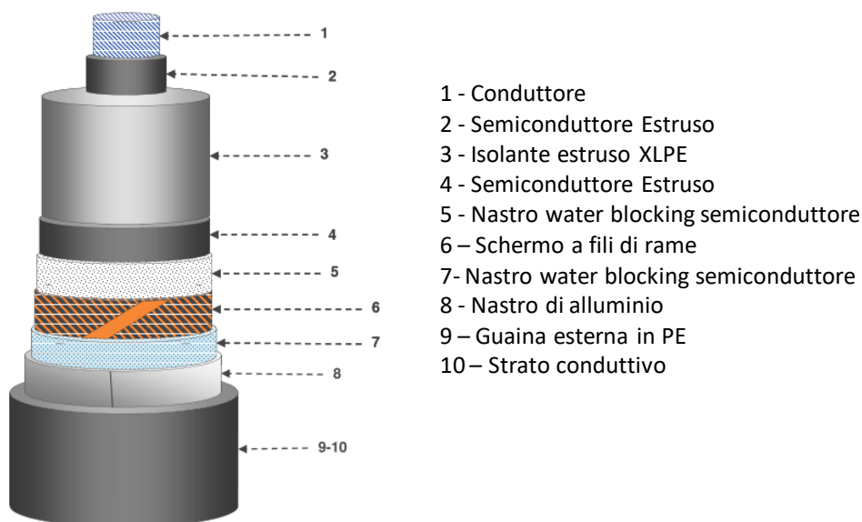
Figura 3-5 - Cavo AT 220 kV tipo ARE4H1H5E 200/345kV
