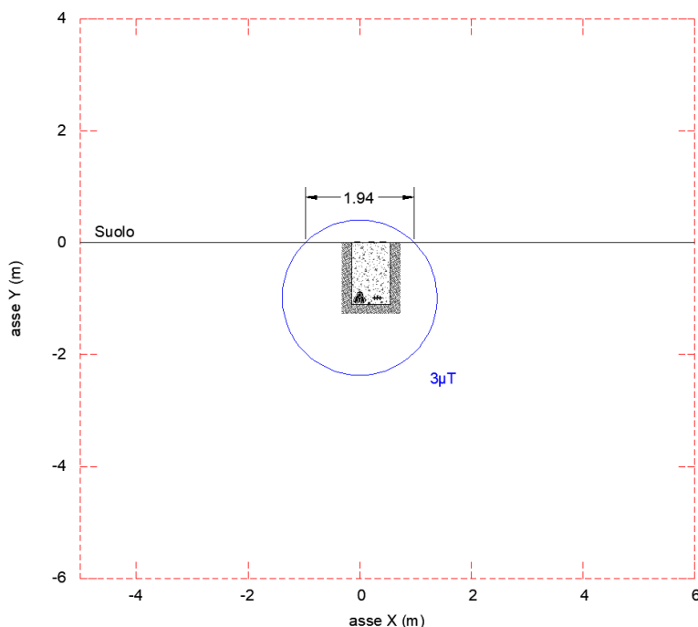
Figura 5-2 - Curva Equilivello 3 \mu T – 1 terna di cavi MT
