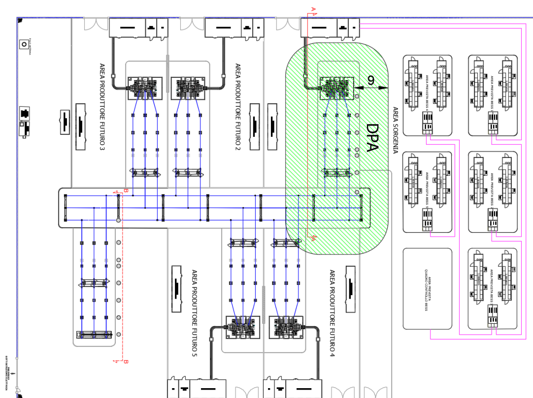
Figura 7-1 - DPA (in m) per lo stallo trasformazione nella SSE Utente 220/30 kV
