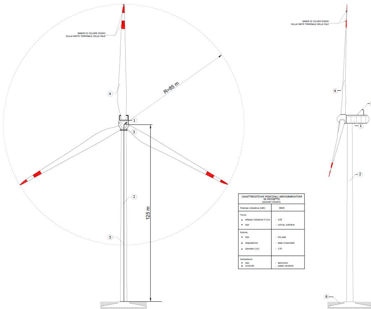
Figura 3-2 – Aerogeneratore tipo SG 6.6-170 altezza al mozzo 125m, e diametro rotore di 170m
