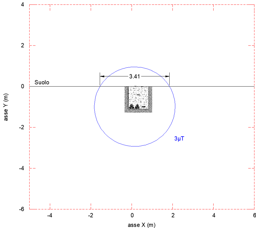
Figura 5-3 - Curva Equilivello 3μT – 2 terne di cavi MT
