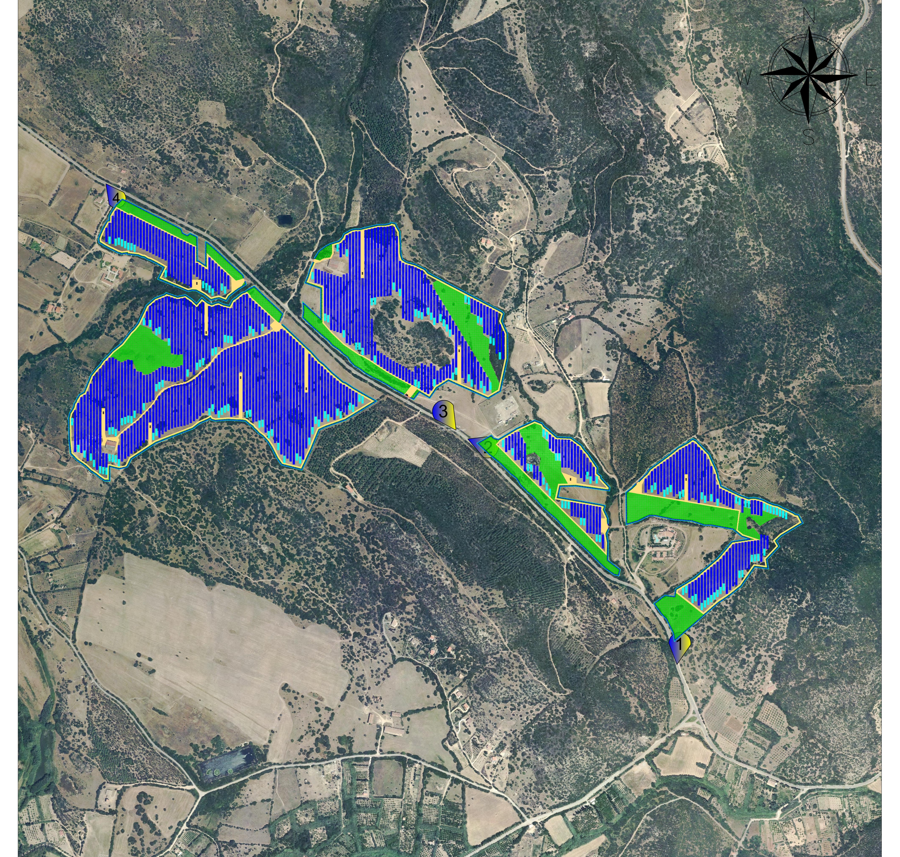
Layout impianto FV_TEULADA su Ortofoto con Punti di Vista
