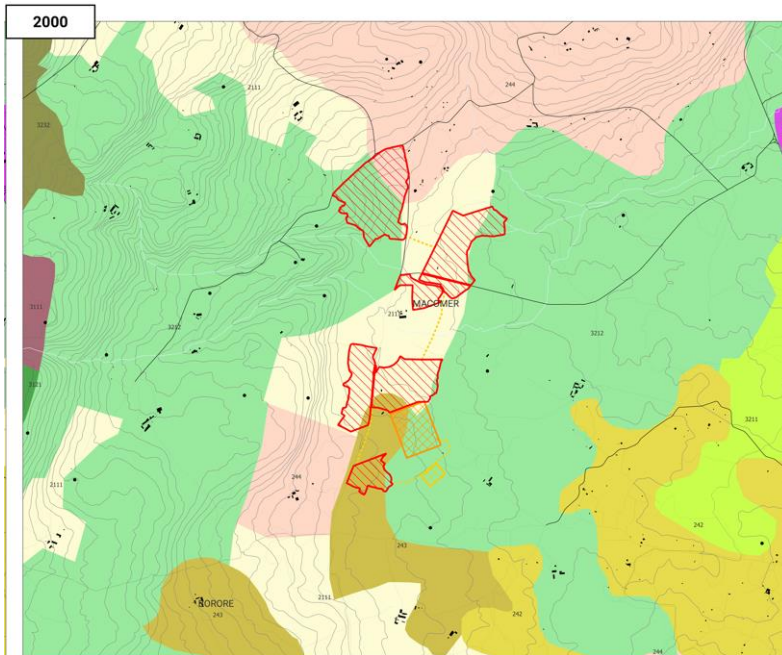
Corine Land Cover anno 2000 e 2006
