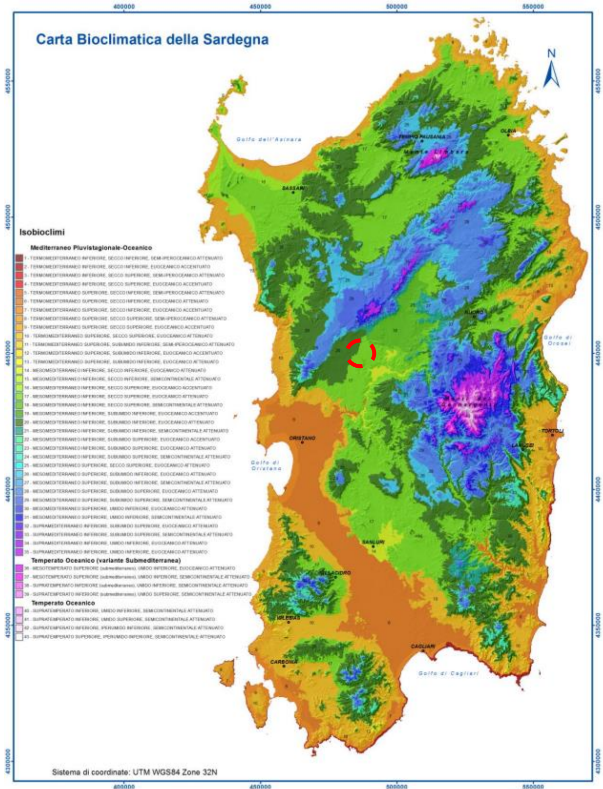
FIGURA 15 - CARTA BIOCLIMATICA DELLA SARDEGNA, CERCHIATA IN ROSSO L'AREA OGGETTO DI STUDIO
