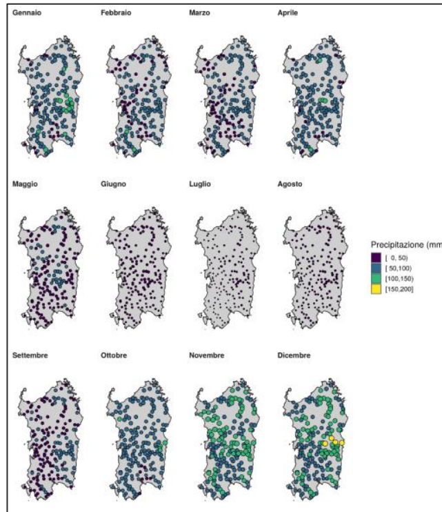
FIGURA 10 - CUMULATI CLIMATOLOGICI MENSILI DI PRECIPITAZIONE PER IL TRENTENNIO 1981-2010
