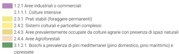
Corine Land Cover anno 2012
