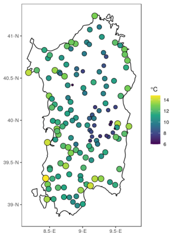
FIGURA 13 - VALORI CLIMATOLOGICI ANNUALI DI TEMPERATURA MINIMA PER IL TRENTENNIO 1981-2010
