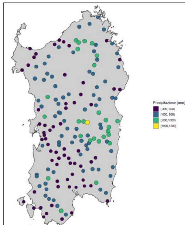
FIGURA 11 - CUMULATI CLIMATOLOGICI ANNUALI DI PRECIPITAZIONE PER IL TRENTENNIO 1981-2010
