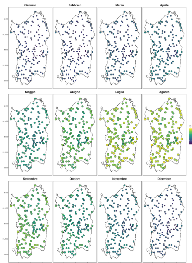
FIGURA 12 - VALORI CLIMATOLOGICI MENSILI DI TEMPERATURA MINIMA PER IL TRENTENNIO 1981-2010
