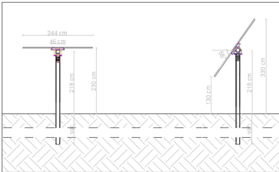
FIGURA 1: TRACKER SOLARE TIPO
