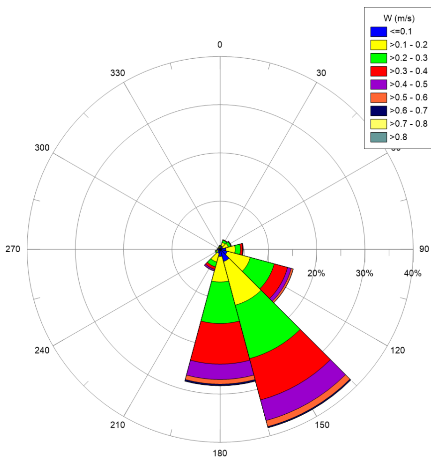
Figura 9.1: Rosa Annuale della Corrente
