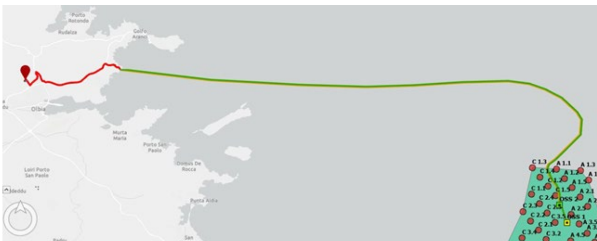
Figura 1.2: Vista Cavidotti Marini e Terrestri del Parco Tibula Energia
