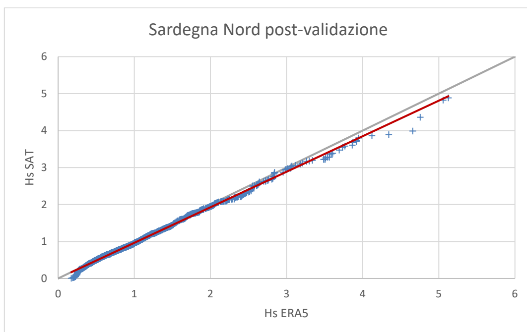
Figura 4.3: Q-Q Plot relativo alla Serie ERA5 non Calibrata (In Alto) e a quella a Valle della Calibrazione effettuata con Dati Satellitari (In Basso)
