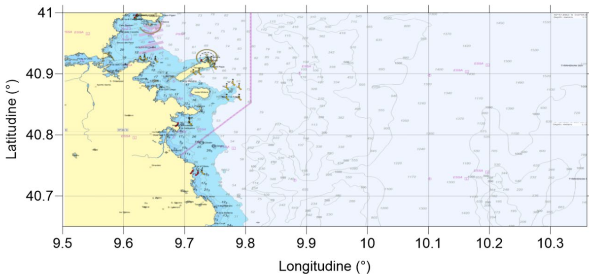
Figura 4.5: Batimetria dell'Area di Studio – IMS (C-MAP)
