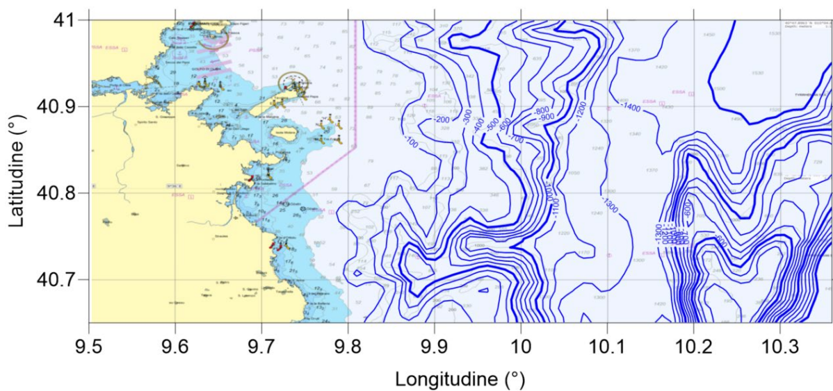
Figura 4.6: Confronto Tra Le Fonti di Dati Batimetrici: IMS (C-MAP) – ETOPO (in blu)
