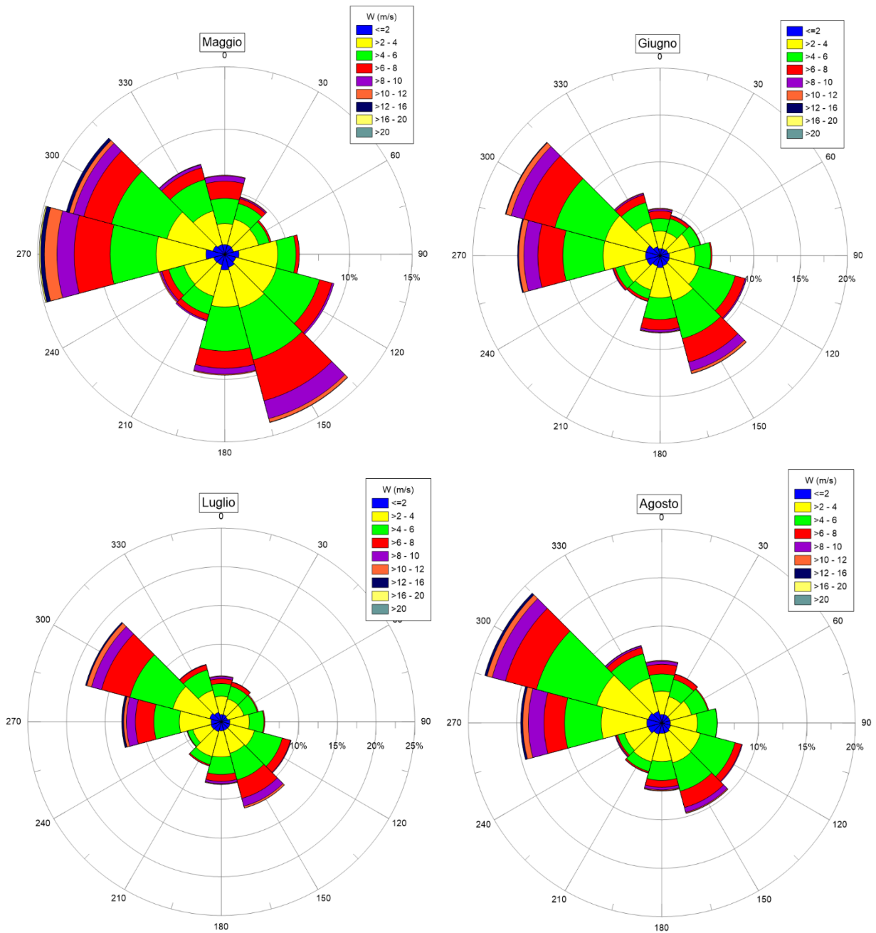
Figura A.2: Rose Mensili del Vento – Maggio, Giugno, Luglio, Agosto - NOAA
