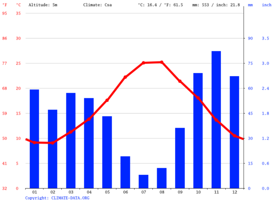
Figura 3.1: Andamento Annuale e Mensile delle Precipitazioni per il Sito di Brindisi
