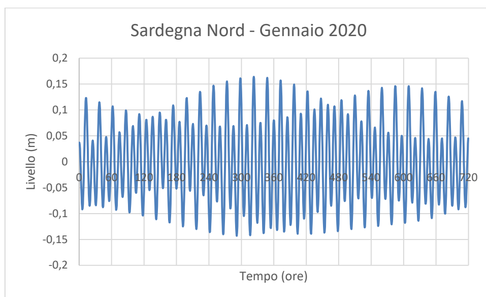
Figura 8.2: Oscillazione del Livello Dovuta alla Marea – Gennaio 2020
