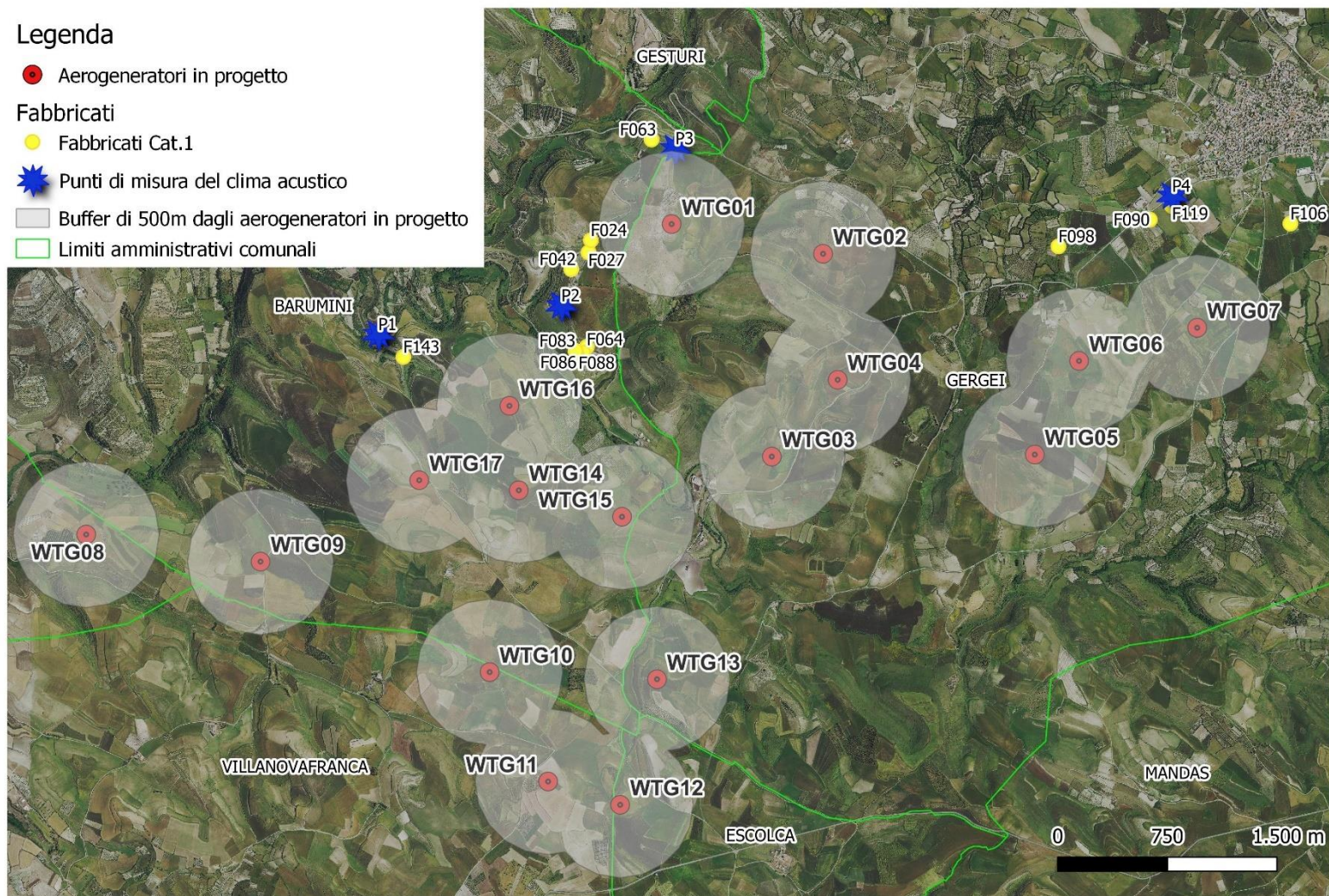
Figura 11.1: Ubicazione delle postazioni di monitoraggio acustico
