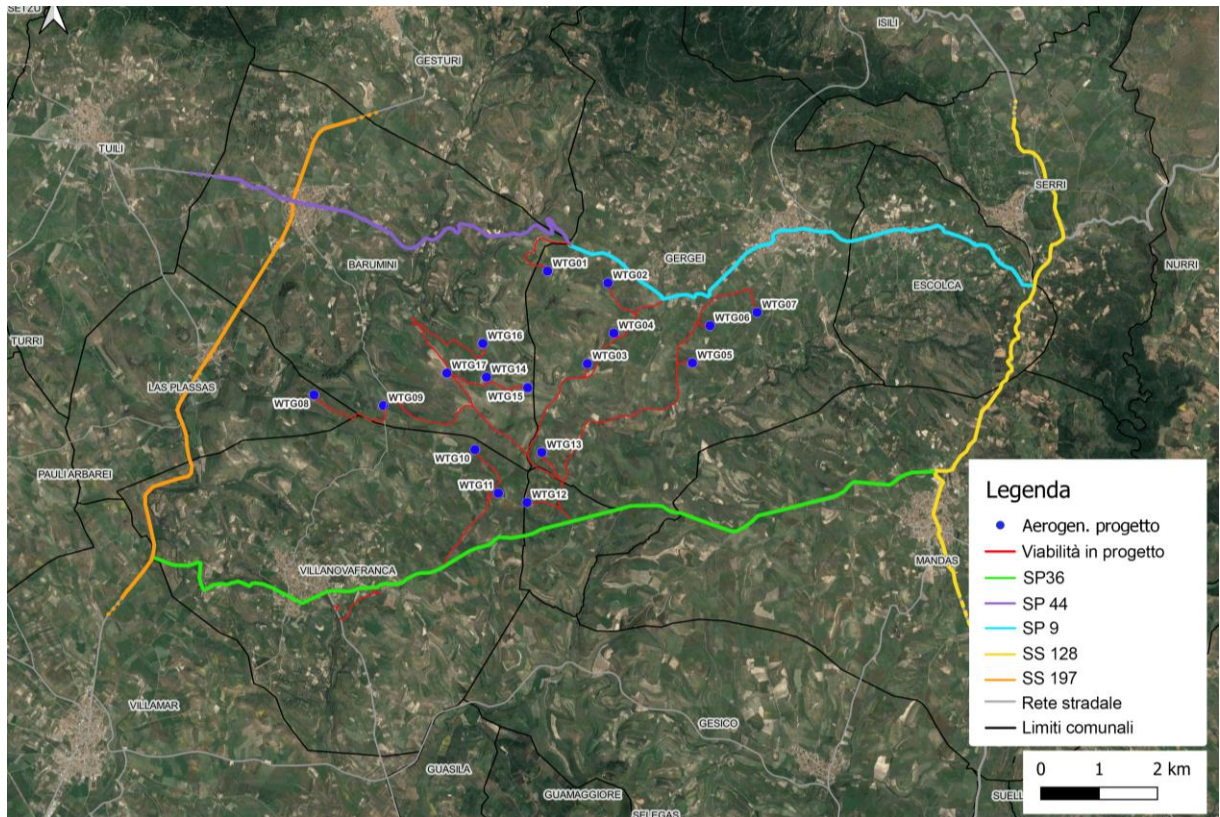
Figura 4.1 – Principali arterie stradali e sistema della viabilità di accesso all’impianto
