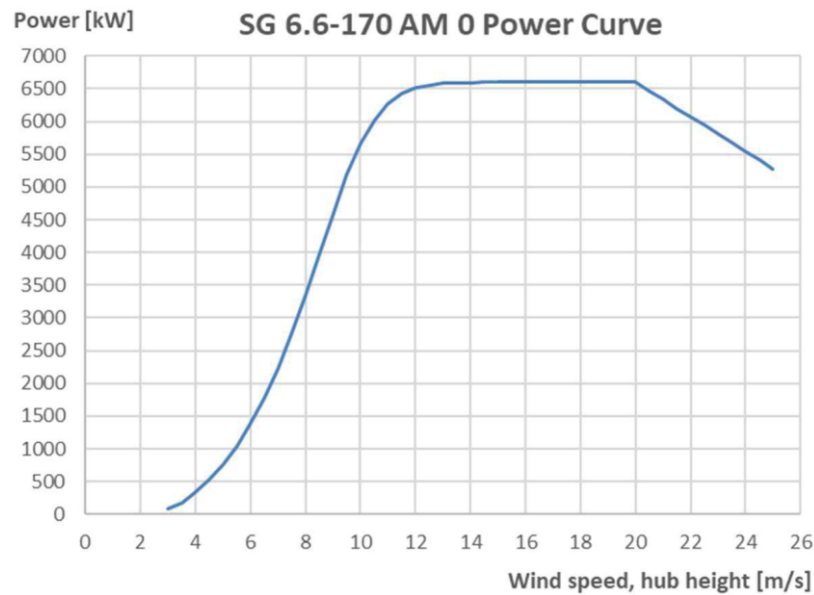
Figura 6.1 - Curva di potenza dell'aerogeneratore di progetto
