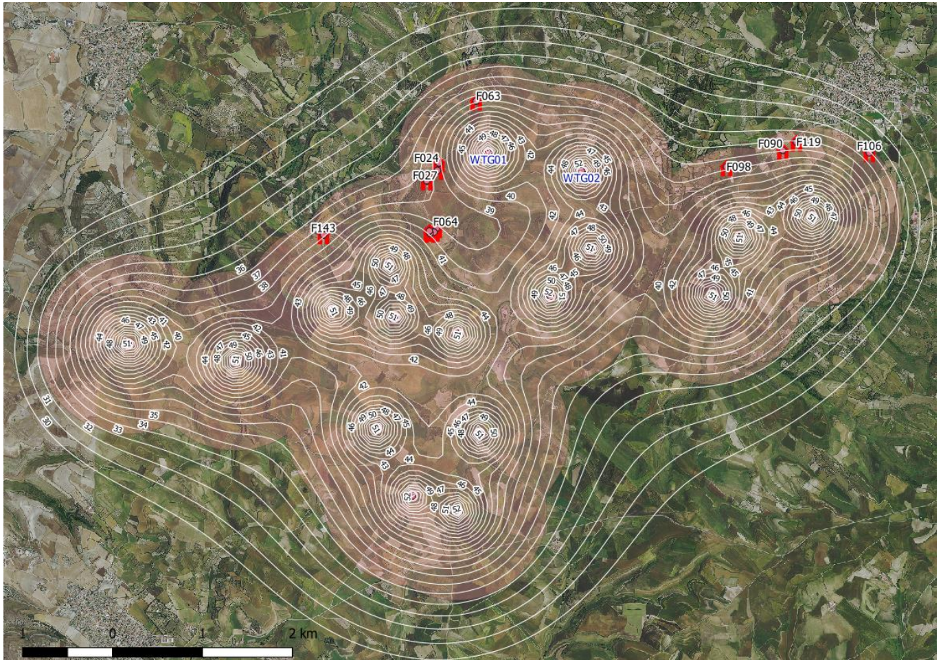
Figura 2.5 – Campo sonoro generato dall'impianto. Si noti come l'isofonica dei 32 dBA sia attestata ad una distanza indicativa di 1.000 m dalle postazioni eoliche in progetto
