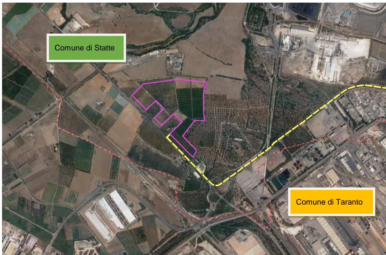
Figura 2-1: Inquadramento territoriale su Ortofoto dall'impianto fotovoltaico annesso all'impianto di produzione di idrogeno
