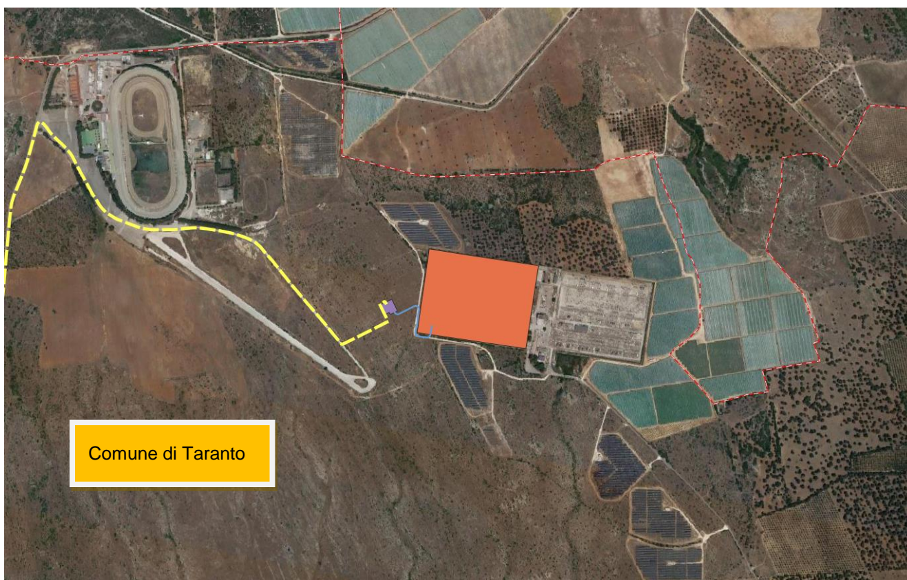
Figura 2-2: Inquadramento territoriale su Ortofoto dell'area interessata dalla Stazione Elettrica TERNA "Taranto N2" (arancione) e dalla Sottostazione Utente (viola)
