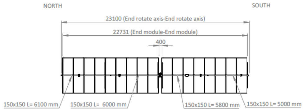
Figura 6-1: Struttura porta pannelli tipo Soltec 2x17
