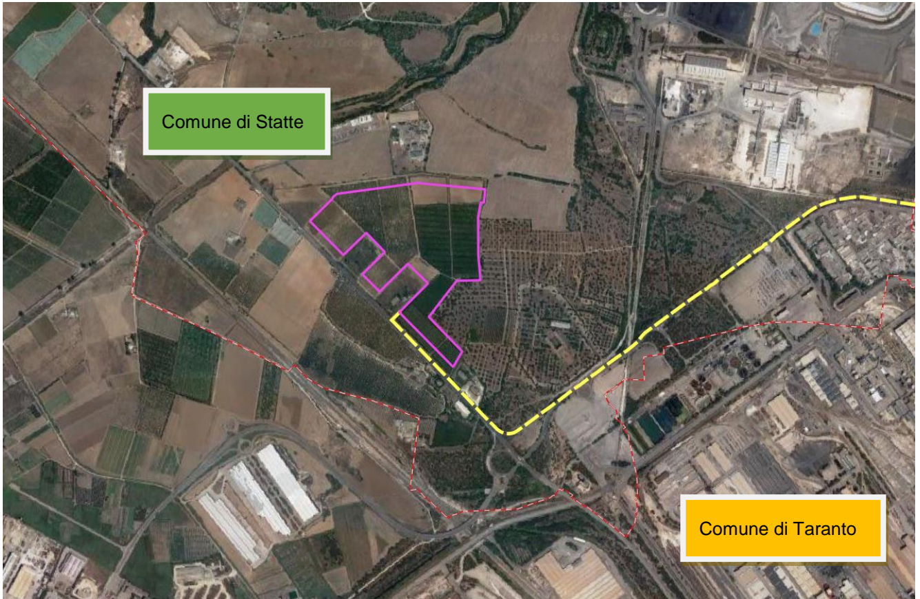
Figura 7-2: Inquadramento territoriale su Ortofoto dall'impianto fotovoltaico annesso all'impianto di produzione di idrogeno
