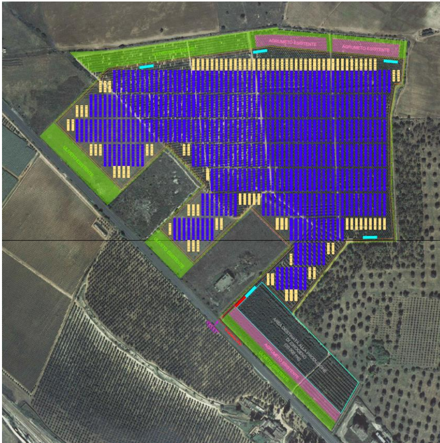
Figura 13-5: Layout di impianto con individuazione delle fasce colturali con funzione schermante
