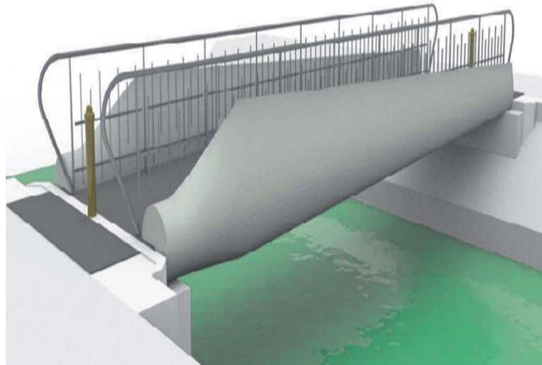
Figura 3: "Analisi e progettazione di un ponte pedonale con pale eoliche e calcestruzzo FRP dismessi", presentato da Raj Suhail al FRPRCS14, Belfast, Regno Unito, 4-7 giugno 2019.
