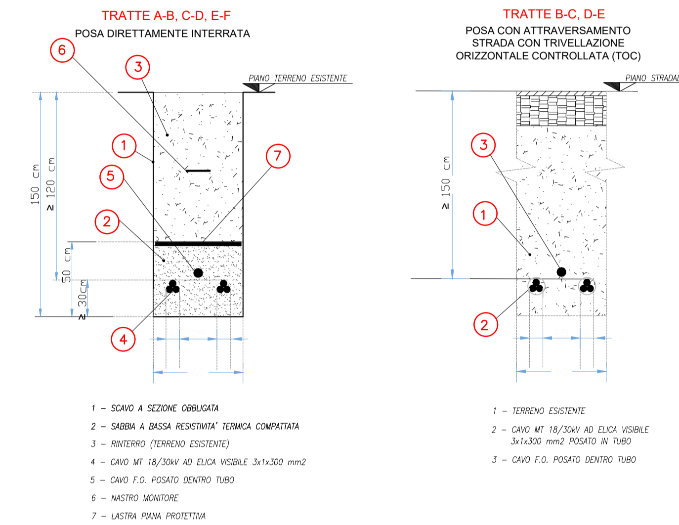
SEZIONI TIPICHE CAVIDOTTO MT - SC. 1:25
