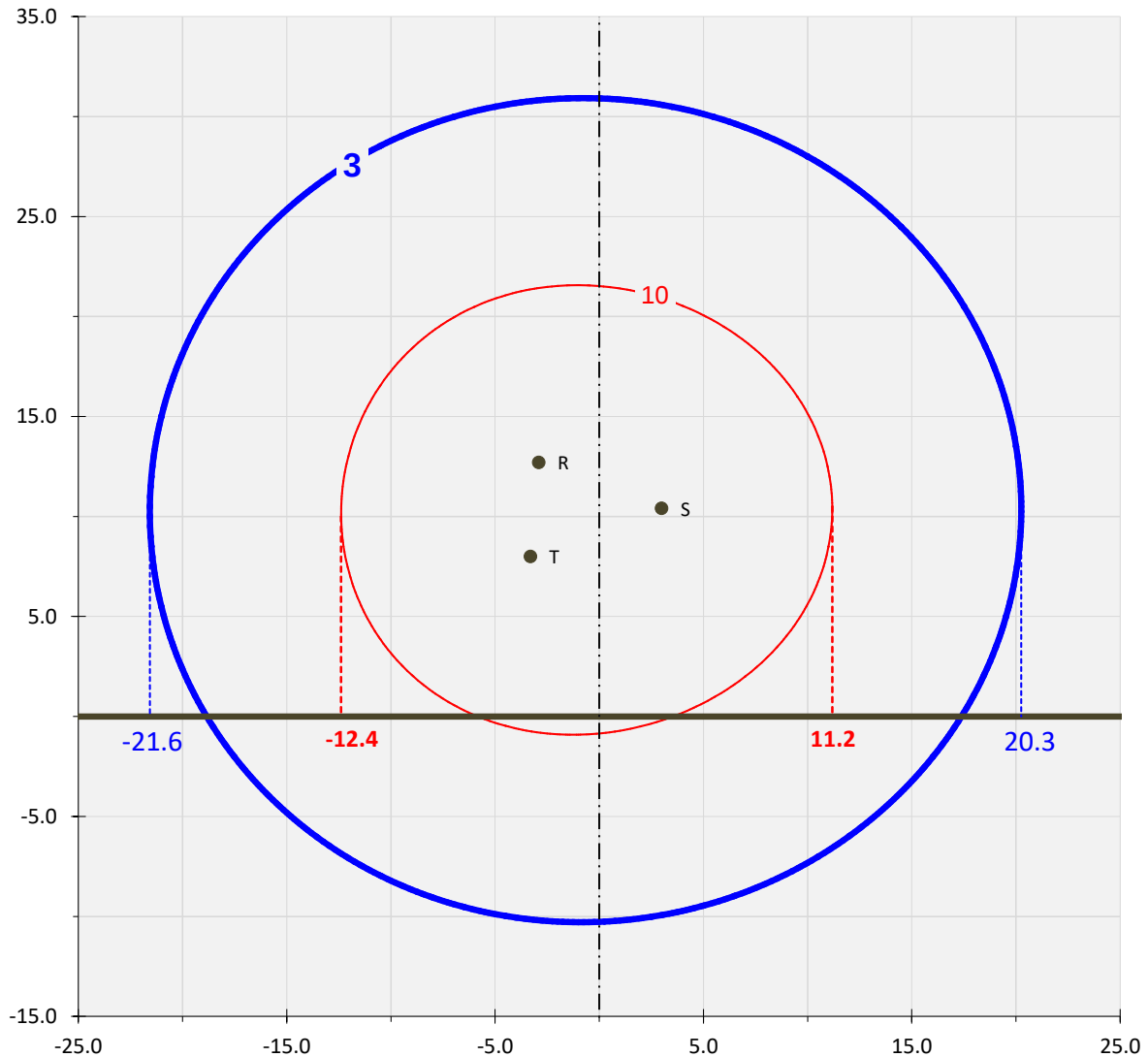
Figura 5.6.2c Curve di Isocampo di Induzione Magnetica in una Sezione Ortogonale all'Asse Linea
