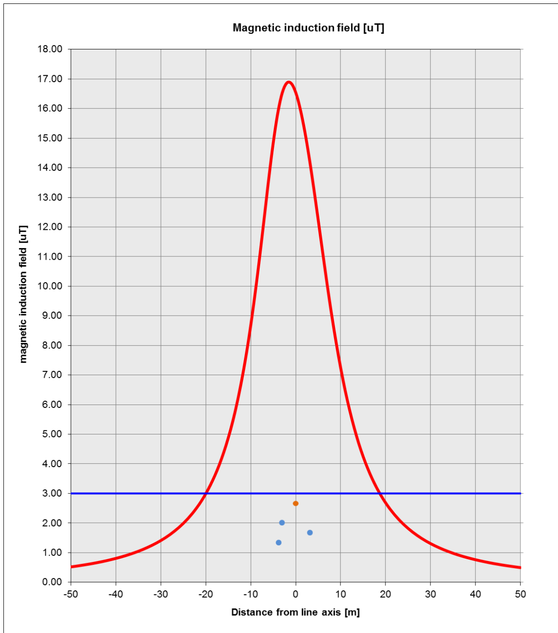
Figura 5.6.2a Andamento dell'Induzione Magnetica in una Sezione Perpendicolare agli Assi della Linea, Calcolata ad 1,5 m dal Suolo nel caso di Franco Minimo (Obiettivo di Qualità pari a 3 microT) – Terna Singola
