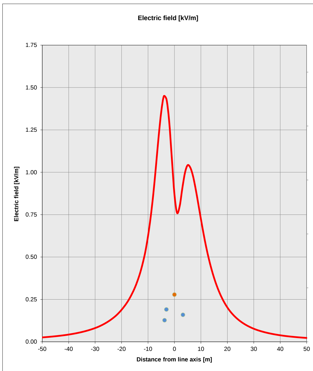
Figura 5.6.2b Andamento del Campo Elettrico in una Sezione Perpendicolare alla Linea, Calcolato ad 1,5 m dal Suolo– Terna Singola (limite di esposizione 5 KV/m)
