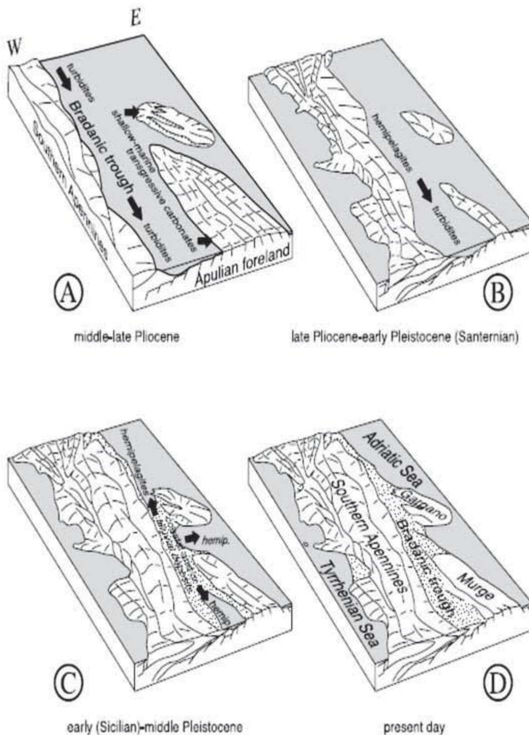
Figura 3.2 - Evoluzione e migrazione dei sistemi deposizionali nell'avanfossa sudappenninica. Da Tropeano et al. , 2002.
