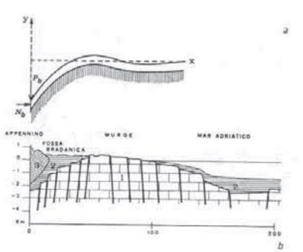
Figura 3.5 - Modello di descrizione del meccanismo di flessione elastica della piattaforma Apula. a) sistema di riferimento per lo studio della flessione di una piastra elastica semi-infinita; b) profilo topografico e geologico schematico dell'Avanpaese Apulo; 1) piattaforma carbonatica Apula; 2) coperture paleogenico-pleistoceniche; 3) coltre alloctona appenninica. Da Ricchetti et al. , 1988.
