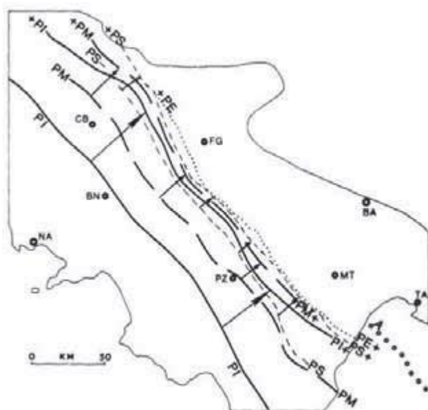
Figura 3.3 - Rappresentazione della migrazione dell'asse depocentrale durante le varie epoche.
