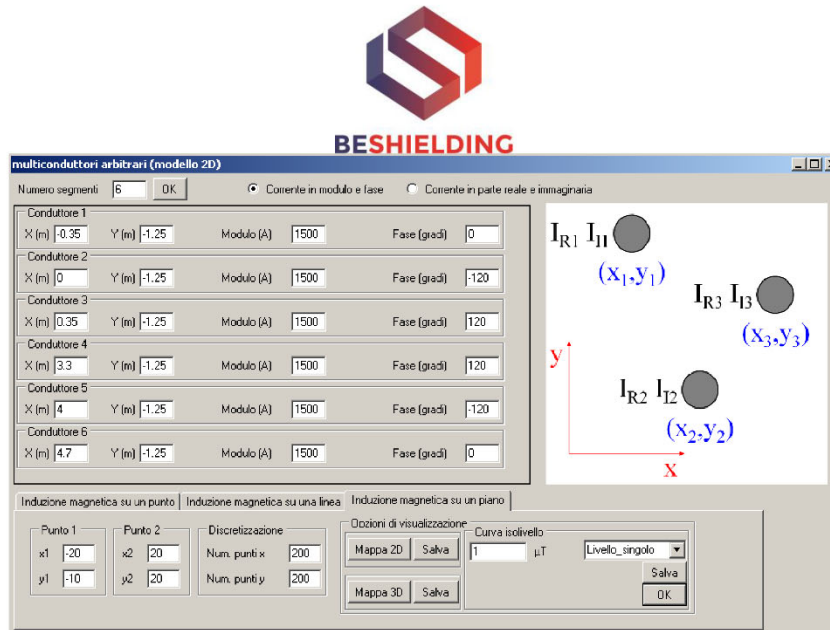
Figura 4: Schermata di ingresso modulo "multiconduttori arbitrari (modello 2D)": dati definizione geometria e sorgenti
