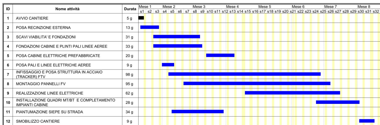
Figura 3.11-1 – Cronoprogramma lavori
