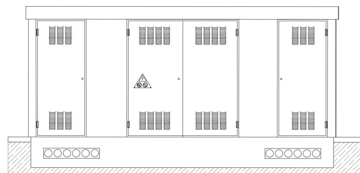
FRONTE
