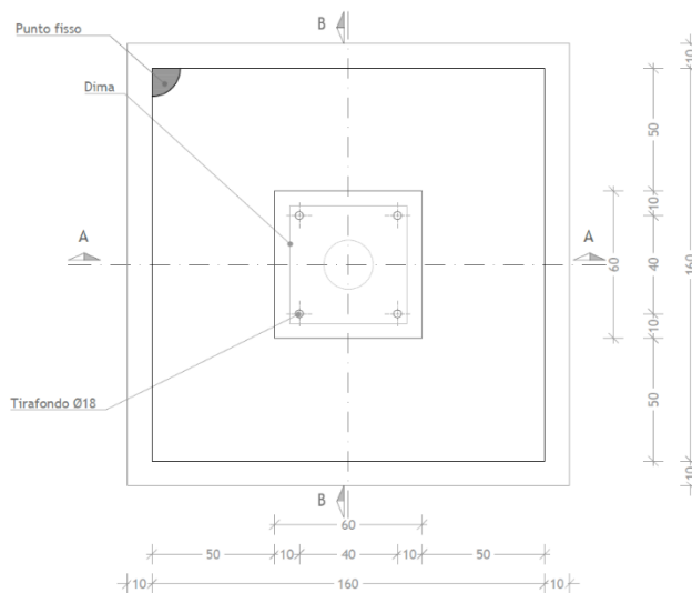
SEZIONE A-A/B-B Scala 1:20
