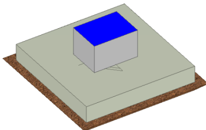
Fig. Vista assonometrica fondazione per terminale cavo AT
