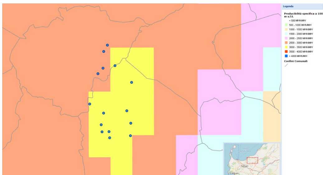
Figura 20 – Estratti Atlante Eolico RSE a 50m, 75m, 100m s.l.t.
