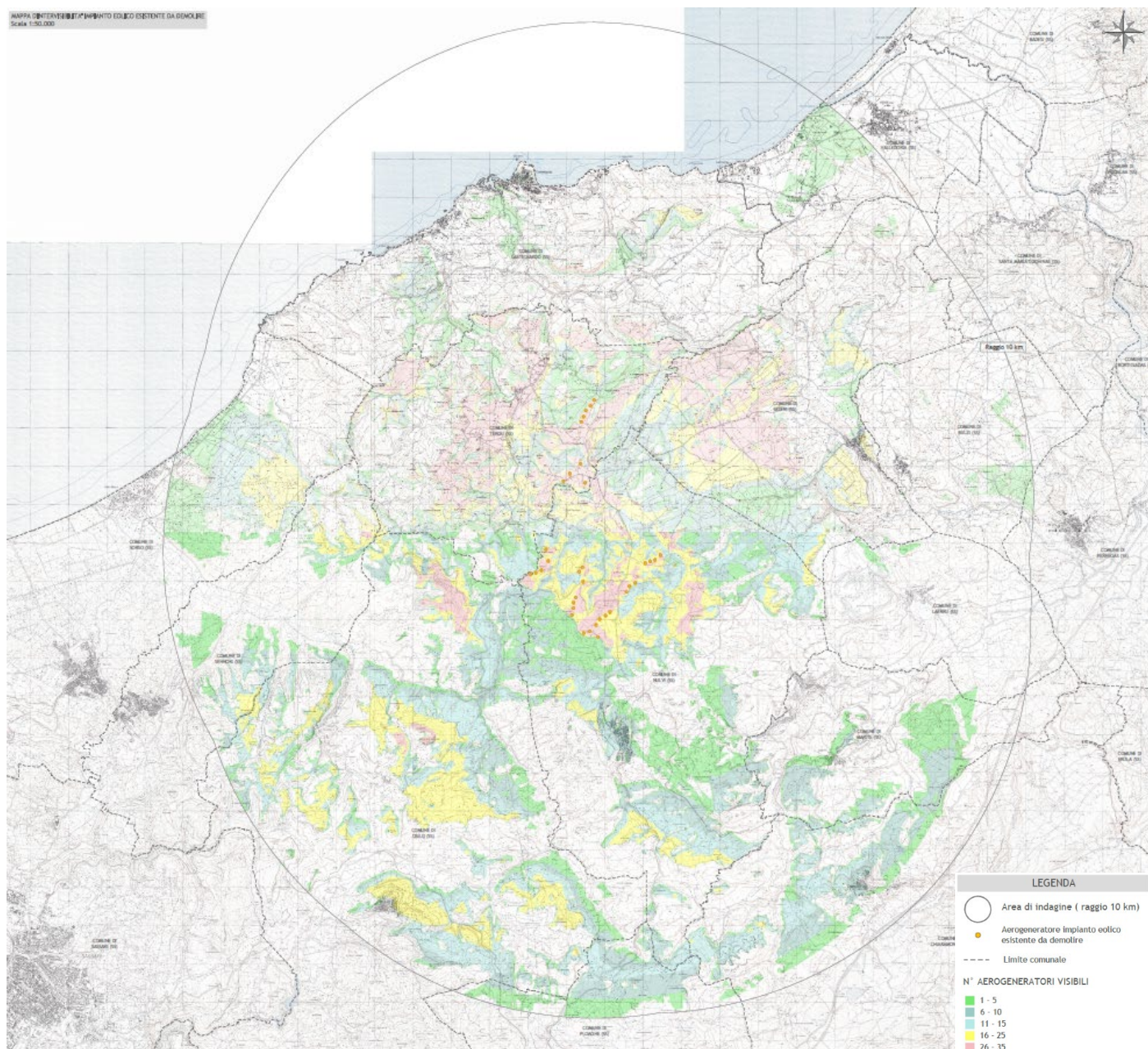
Figura 40 – Stralcio della Mappa d'intervisibilità_Impianto Eolico Esistente
