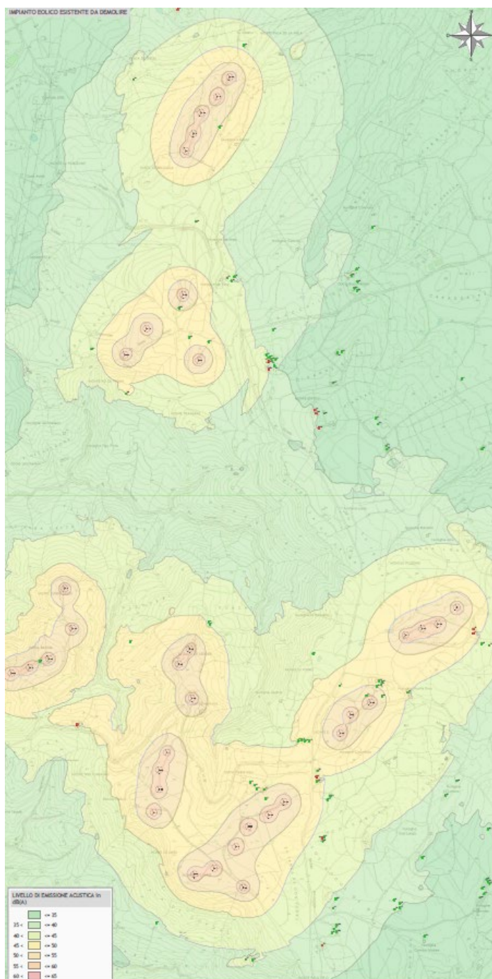
Figura 43 – Livelli di emissione acustica _ Impianto eolico esistente
