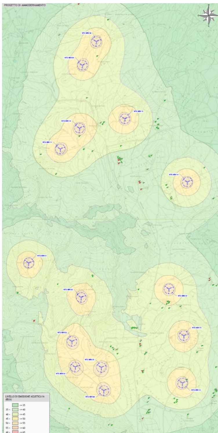
Figura 44 – Livelli di emissione acustica _ Progetto di ammodernamento
