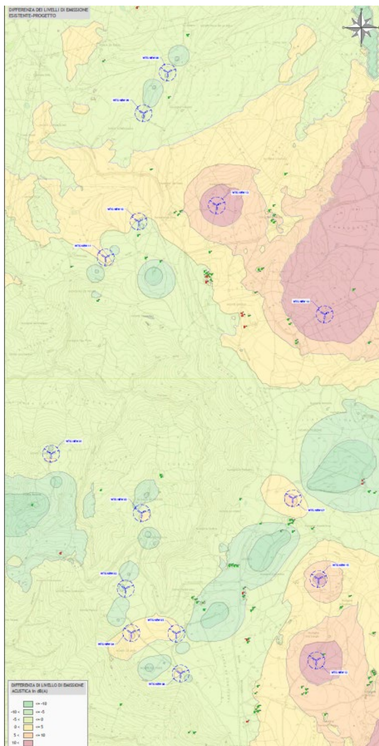
Figura 45 – Differenza dei Livelli di emissione acustica _ Impianto eolico esistente/Progetto di ammodernamento
