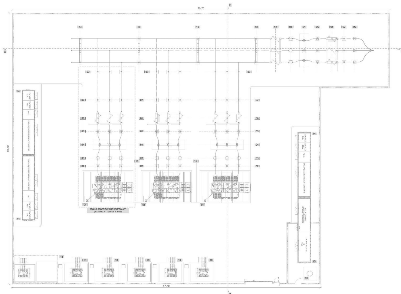
Figura 27 – Planimetria Elettromeccanica
