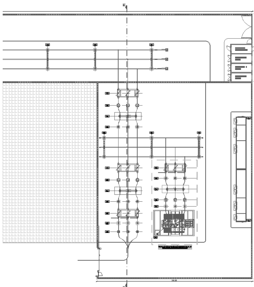
Figura 31 – Planimetria Elettromeccanica
