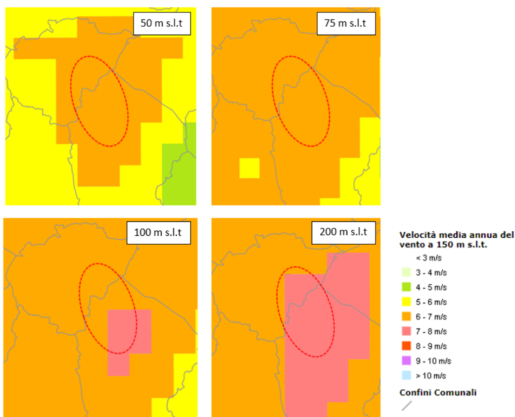
Figura 35 – Velocità media annua del vento a 50, 75, 100 e 200 m s.l.t./s.l.m. Fonte AtlaEolico, consultabile liberamente a
