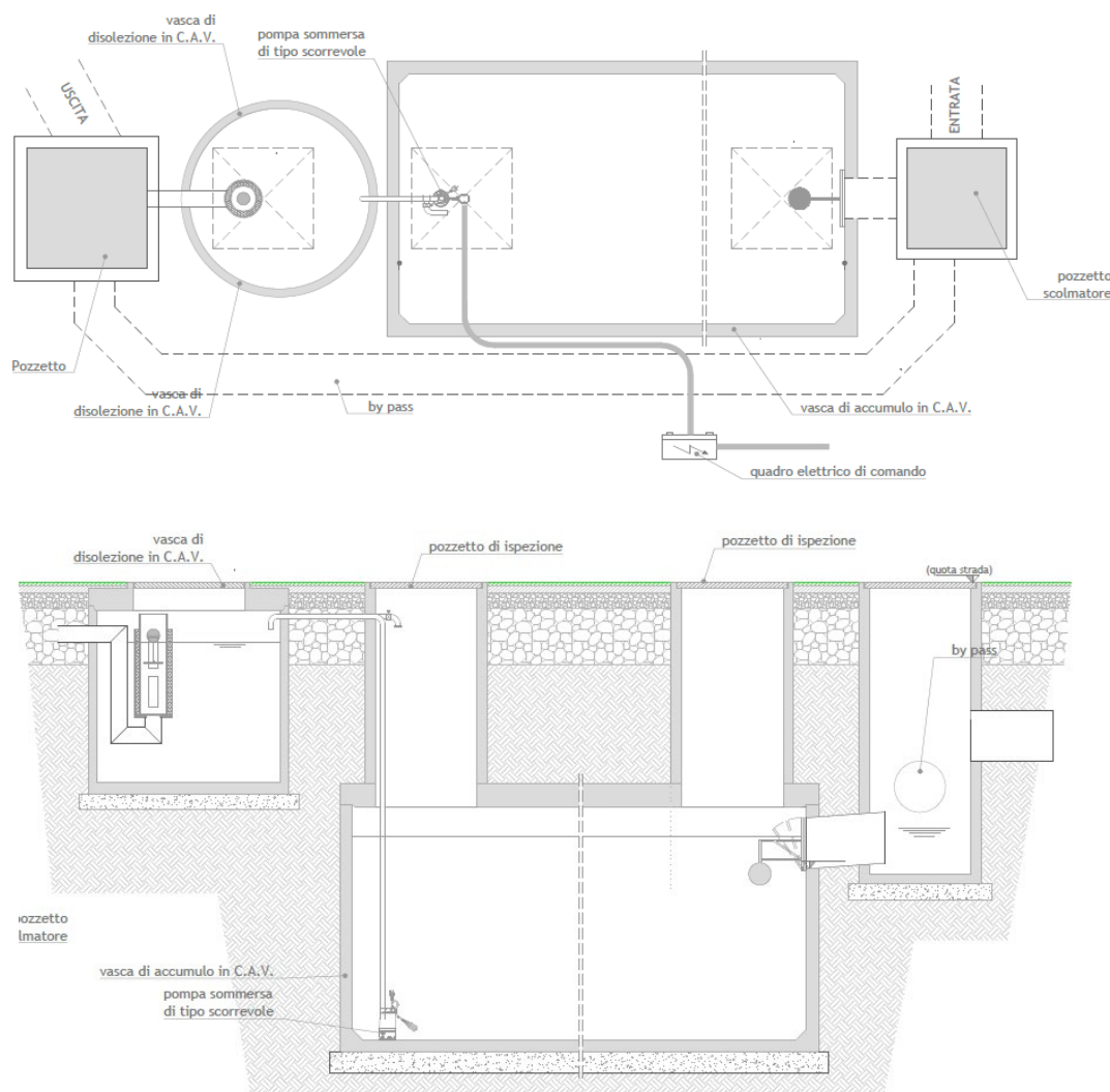
Figura 30 - Schema tipo sistema di trattamento acque di dilavamento
