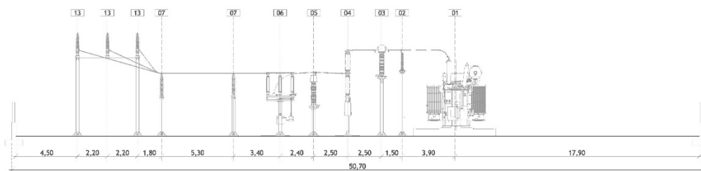
Figura 28 – Sezioni Elettromeccaniche
