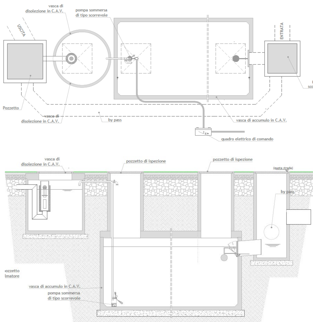
Figura 34 - Schema tipo sistema di trattamento acque di dilavamento
